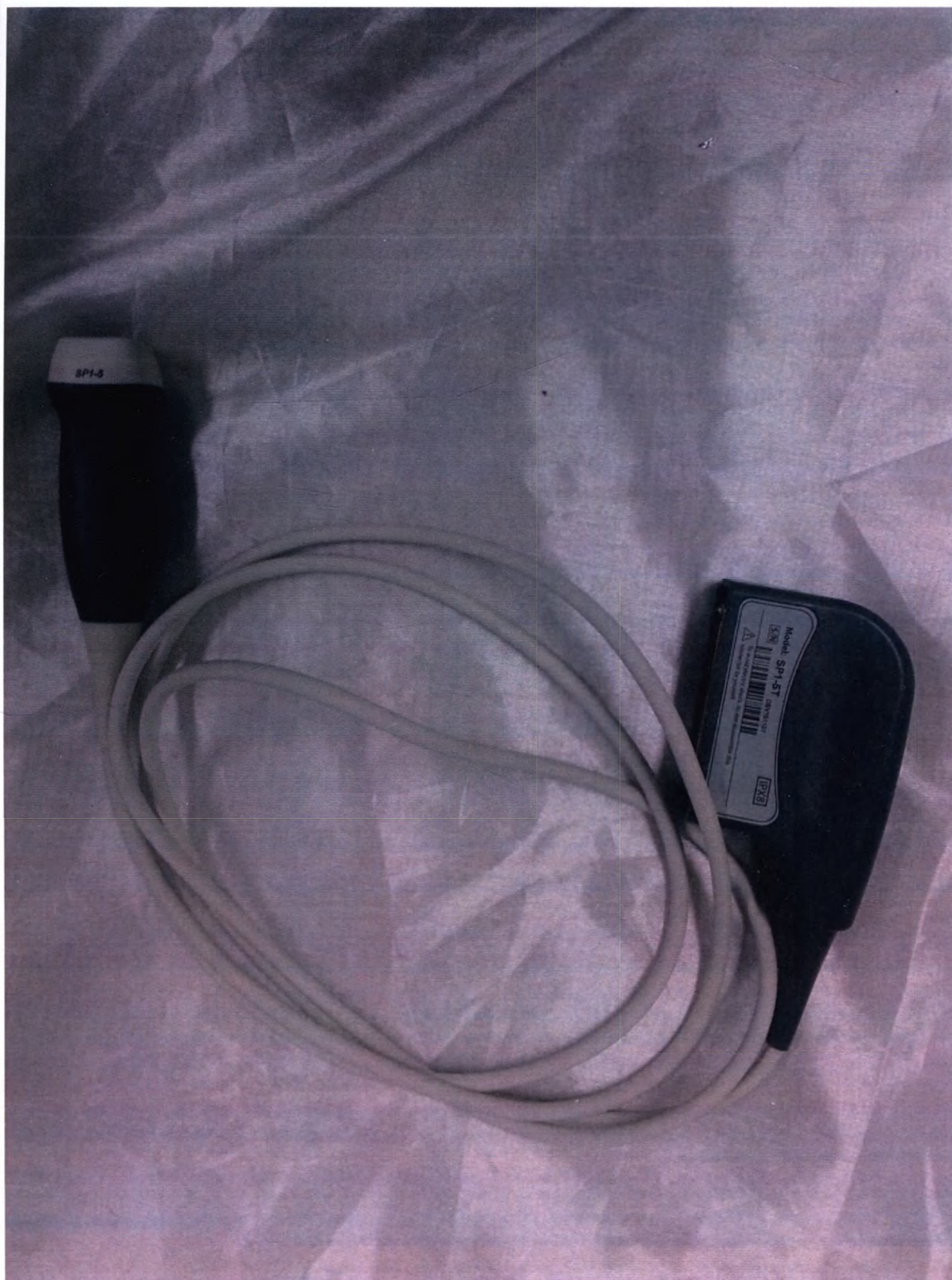
Фото 16. Датчик ультразвуковой секторный монокристаллический серии SP "SP1-5T"
