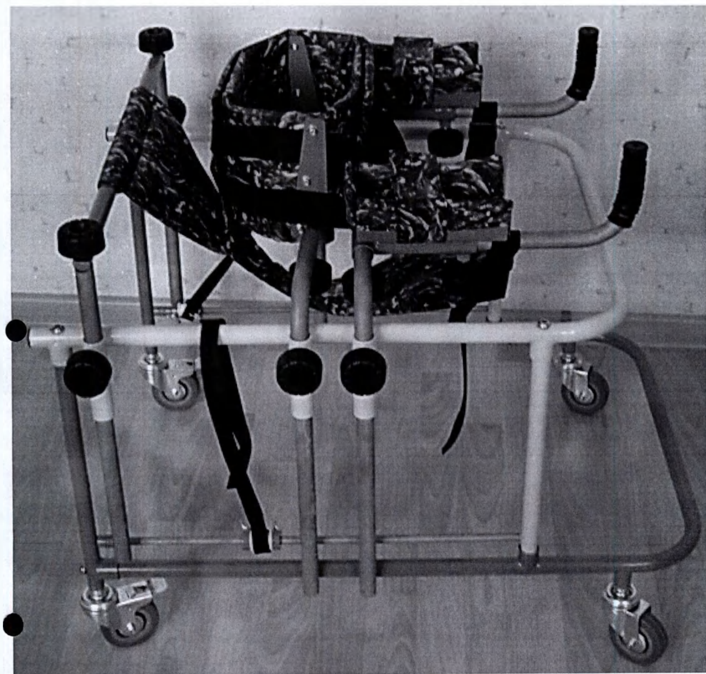
Ходунки Ortonica ХК800 (размер S) по ТУ 32.50.22-005-66445146-2017
