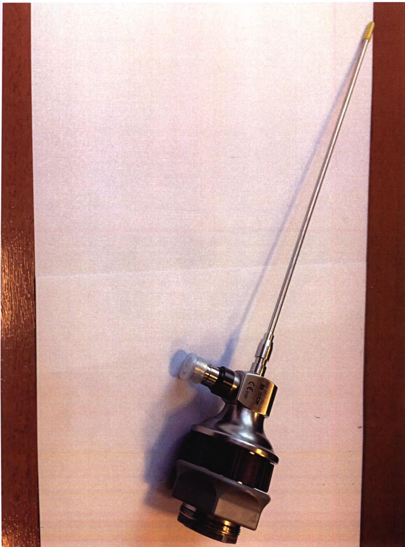
Артроскоп Precision IE 4K с С-образным креплением 2,9 мм x 30°, 200 мм, с фиксатором Speed-Lock
