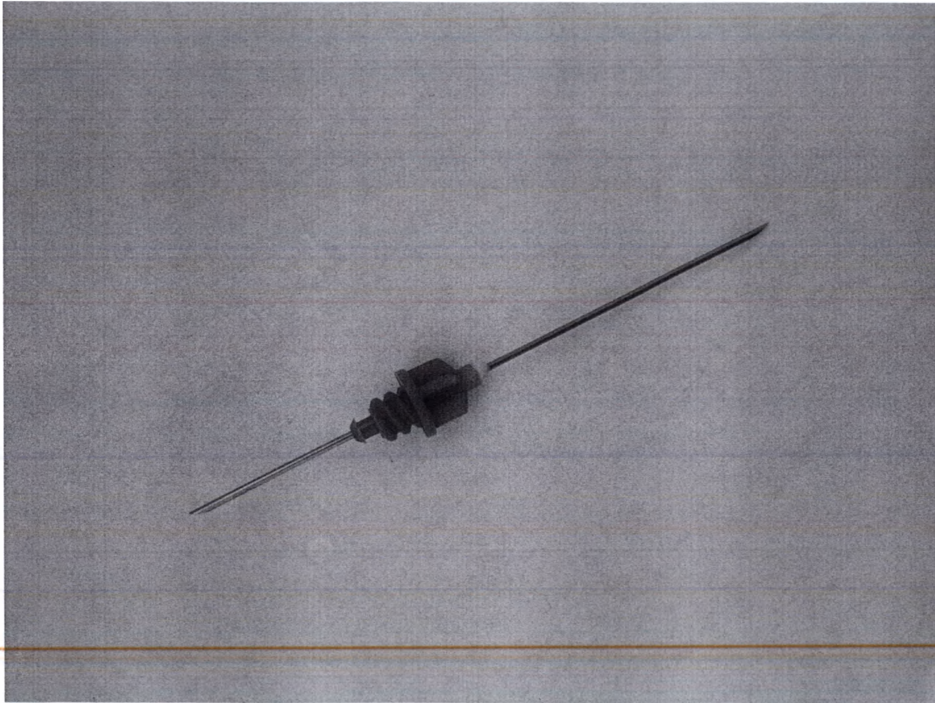
Игла медицинская двухсторонняя для забора венозной крови 0,8x25 без резинового колпачка на дистальном конце.
