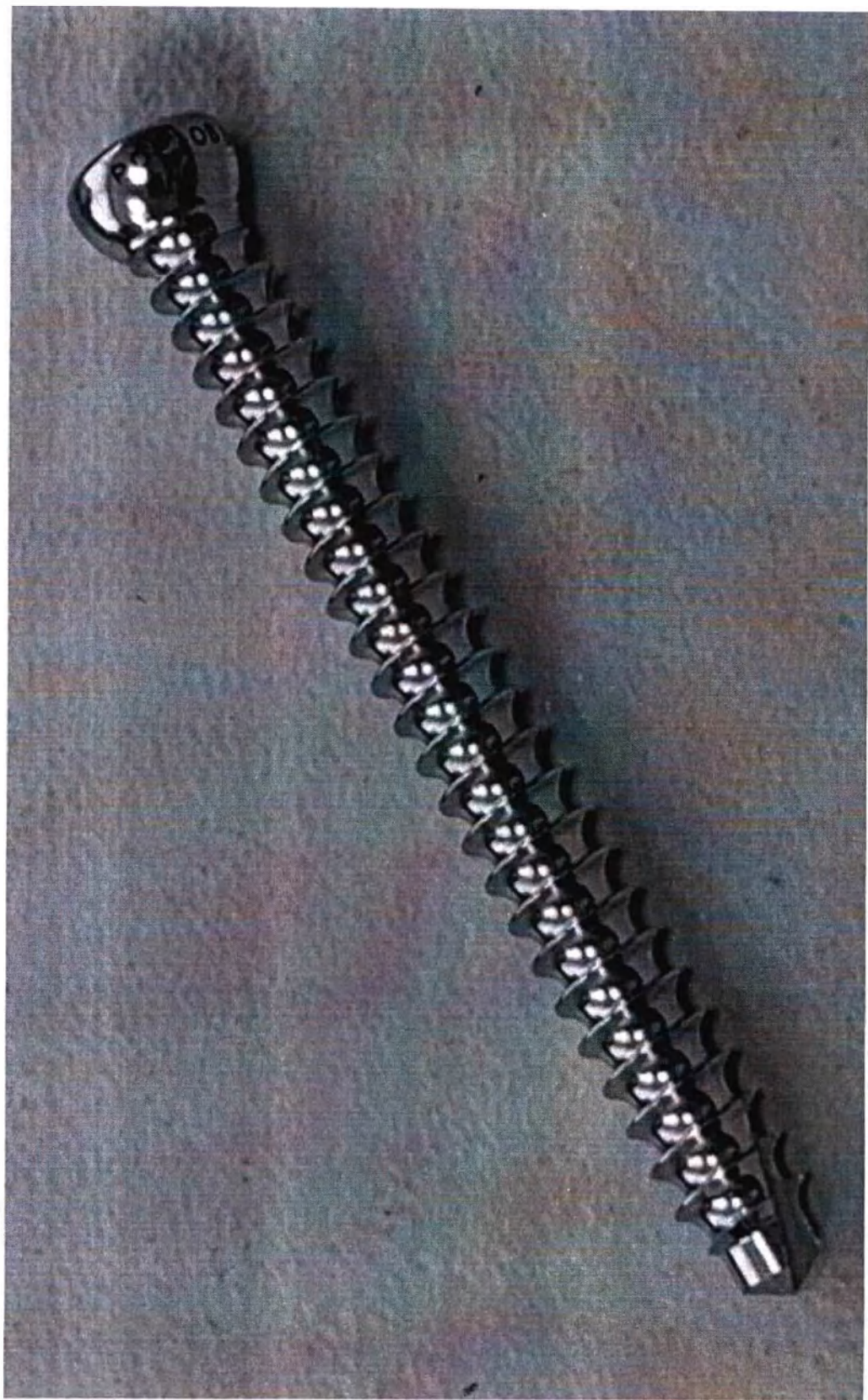
12. Полиаксиальный компрессионный винт, \varnothing 3,5 мм X L = 36 мм, POP-OB35-36
