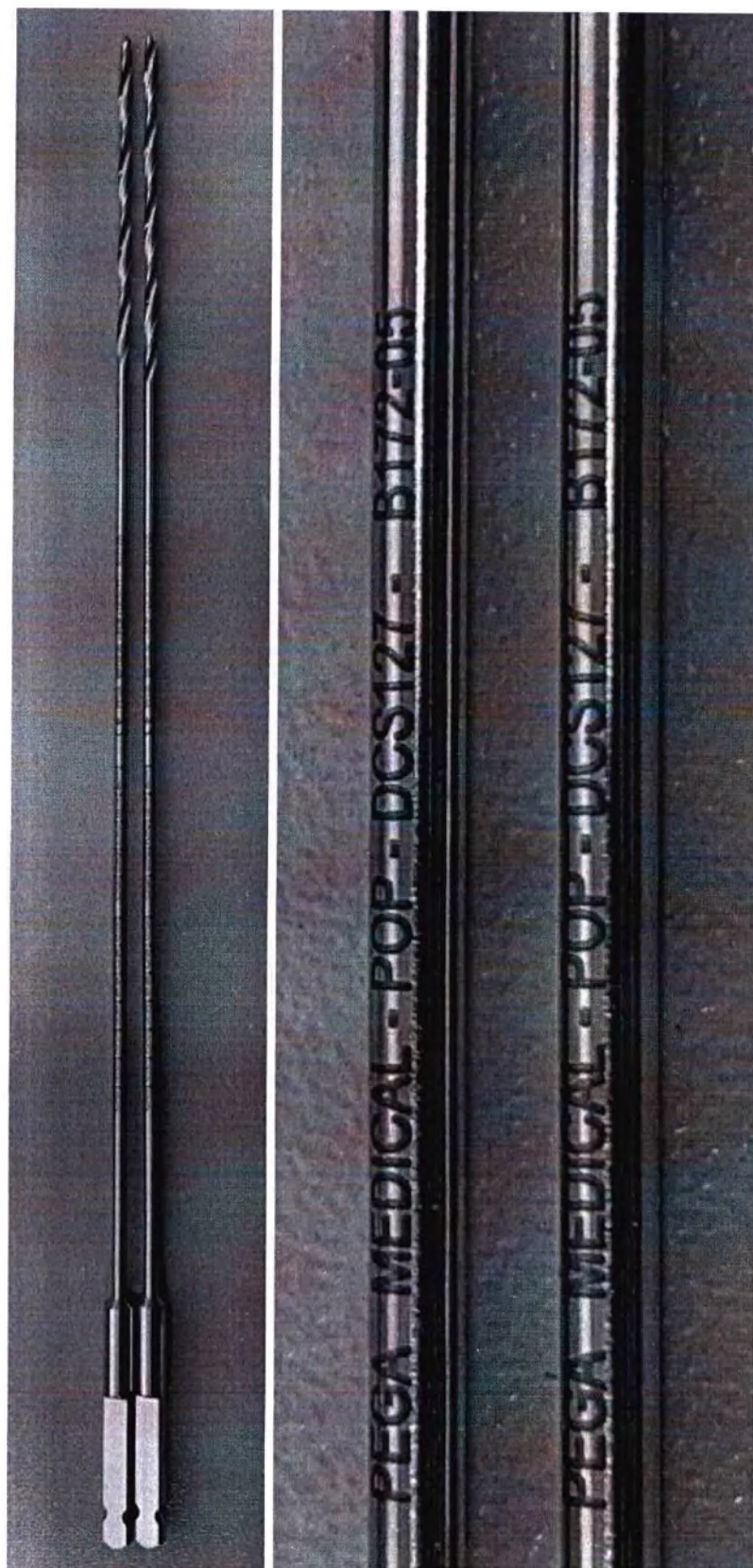
18. Сверло кортикальное, Ø2,7 мм, POP-DCS127
