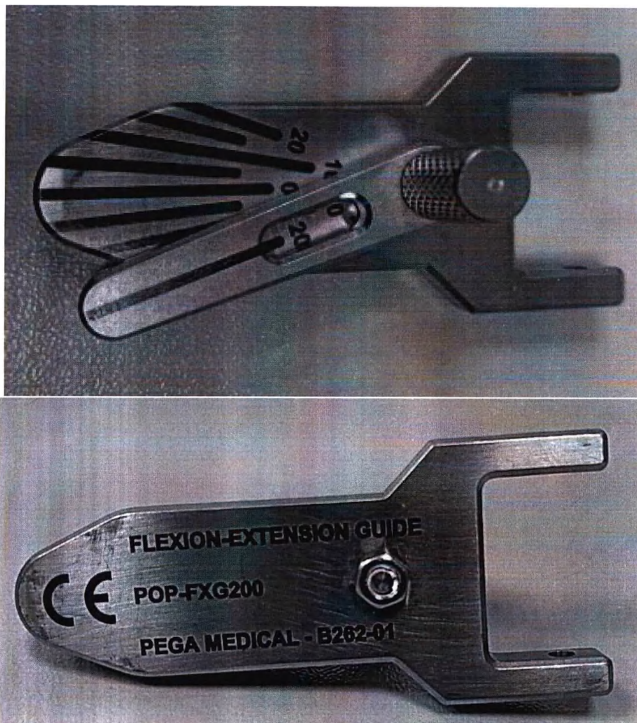
15. Направляющая для сгибания/разгибания, POP-FXG200
