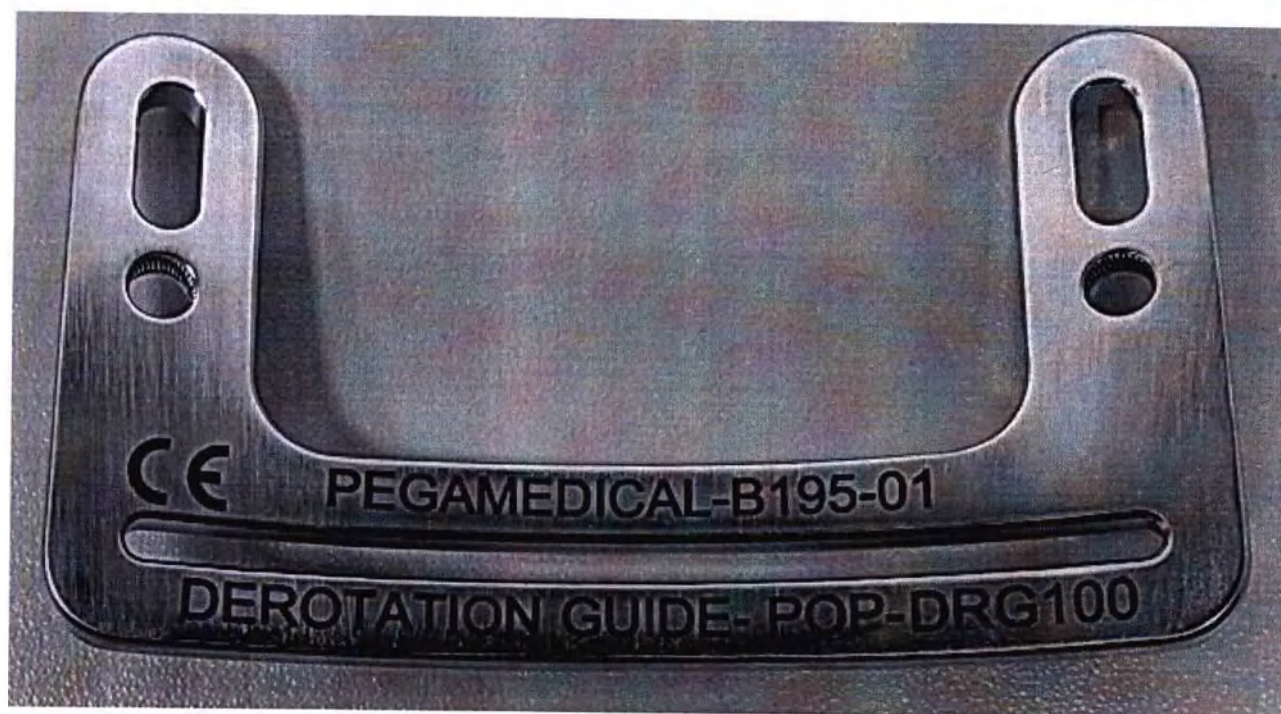
28. Деротационная направляющая, POP-DRG100
