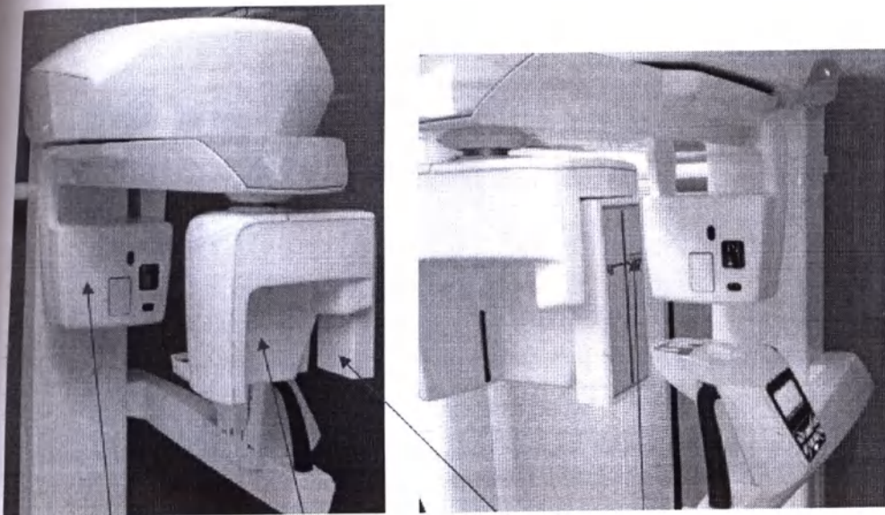
Фото 6. Тубус рентгеновской трубки, детектор СВЗД и модуль детектора.
