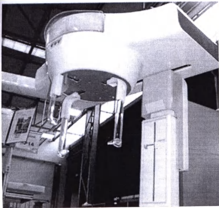
Фото 7. Цефалометрическая группа с устройством для фиксации пациента и сенсором СЕРН.
