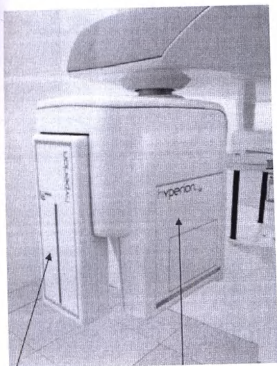
Фото 5. Детектор СВЗД и модуль детектора.
