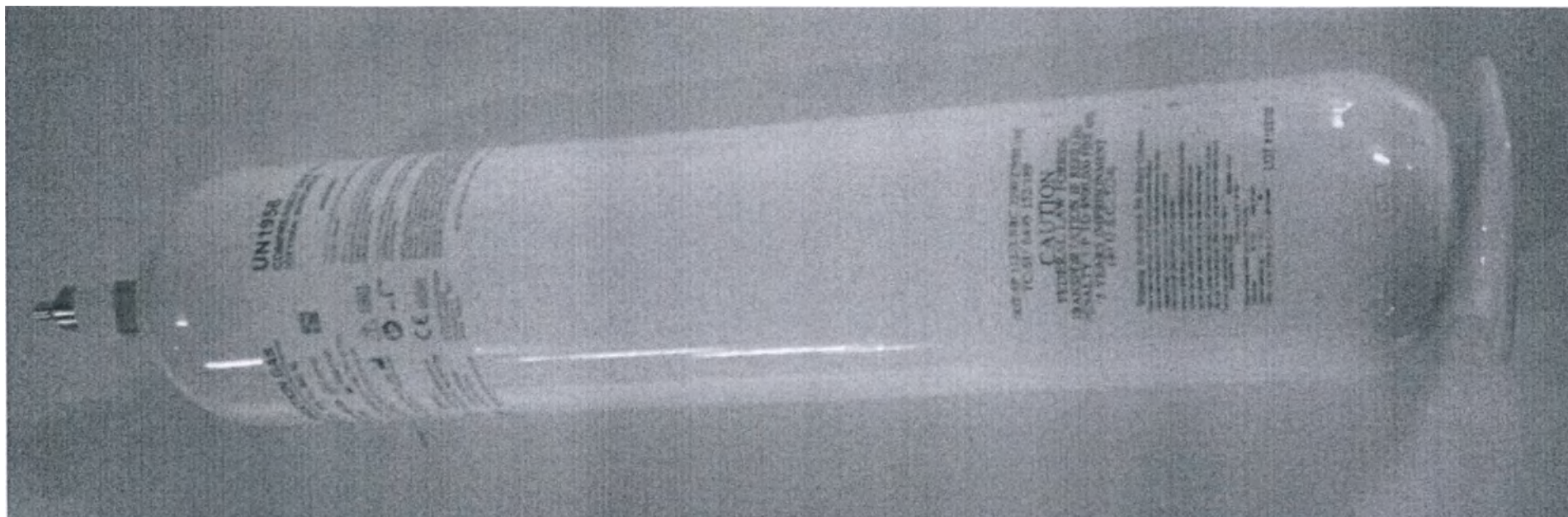
Баллон с калибровочной газовой смесью (16%O 2 , 5%CO 2 , N 2 ост.)
