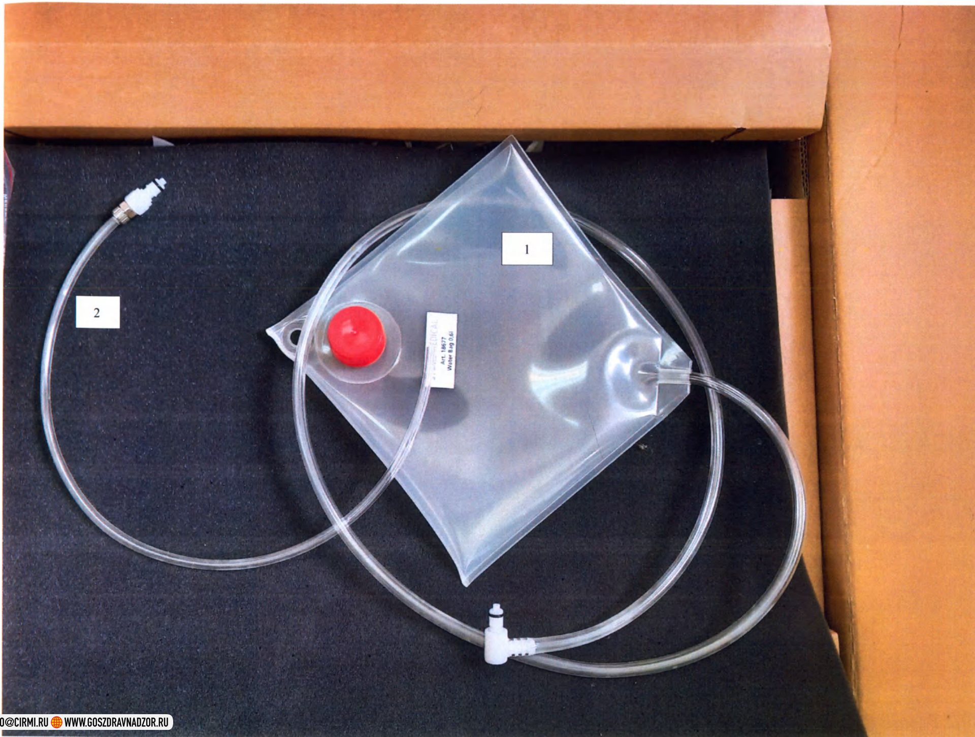
Фото 12. (1) Мешок для замены воды; (2) Трубка для промывки/перетока воды:
