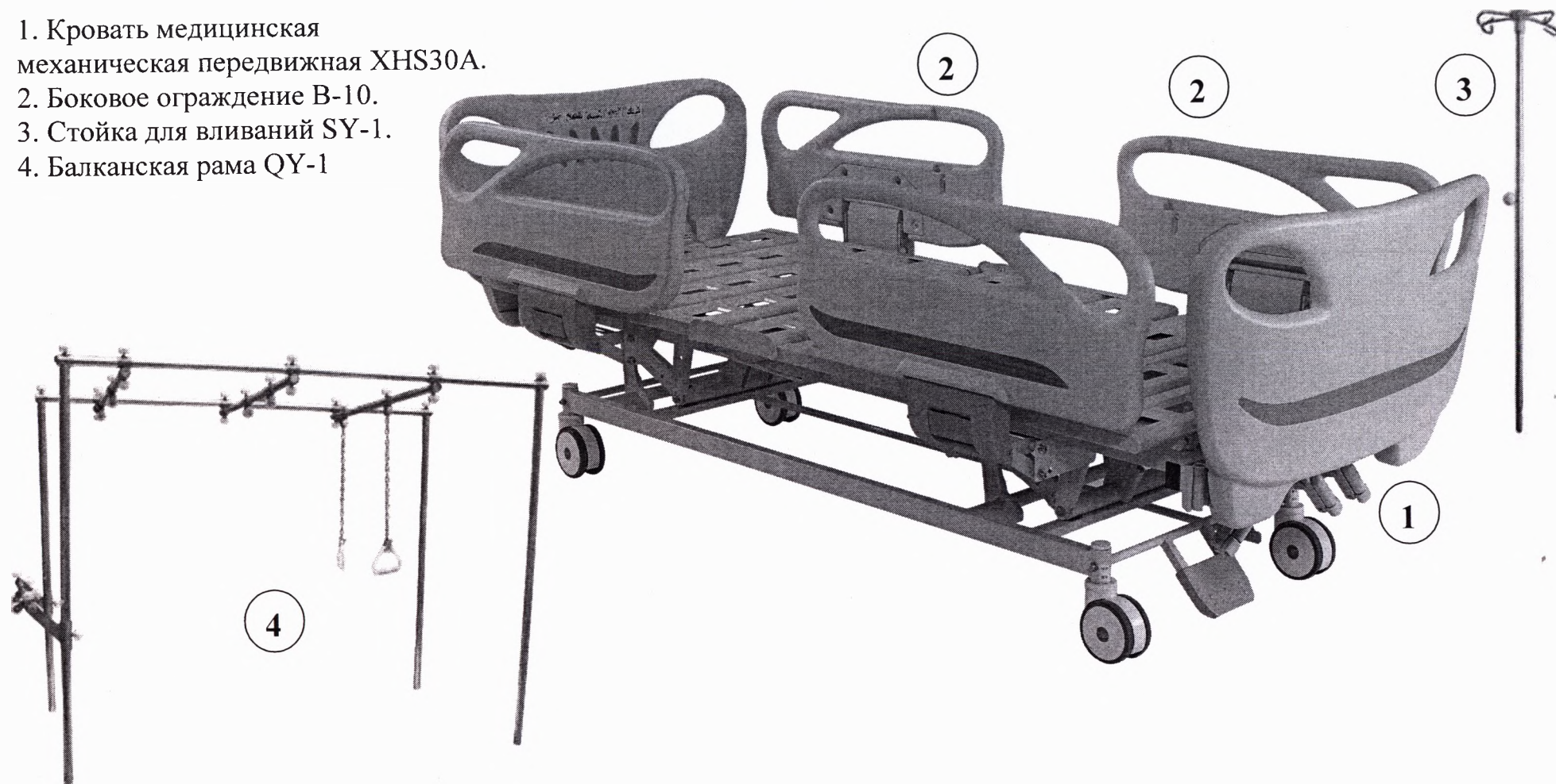
Кровать медицинская механическая передвижная 4-х секционная XHS30A: Вариант исполнения XHS30A-00, с боковыми ограждениями и стойкой для вливаний. Вариант исполнения XHS30A-02, с боковыми ограждениями и балканской рамой.
