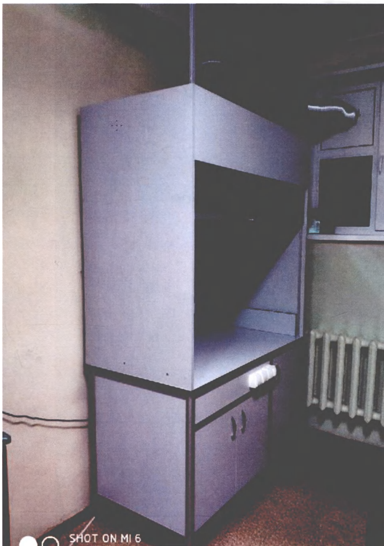
Шкаф лабораторный химический вытяжной с бактерицидной лампой (Арт. ВШ-004)
