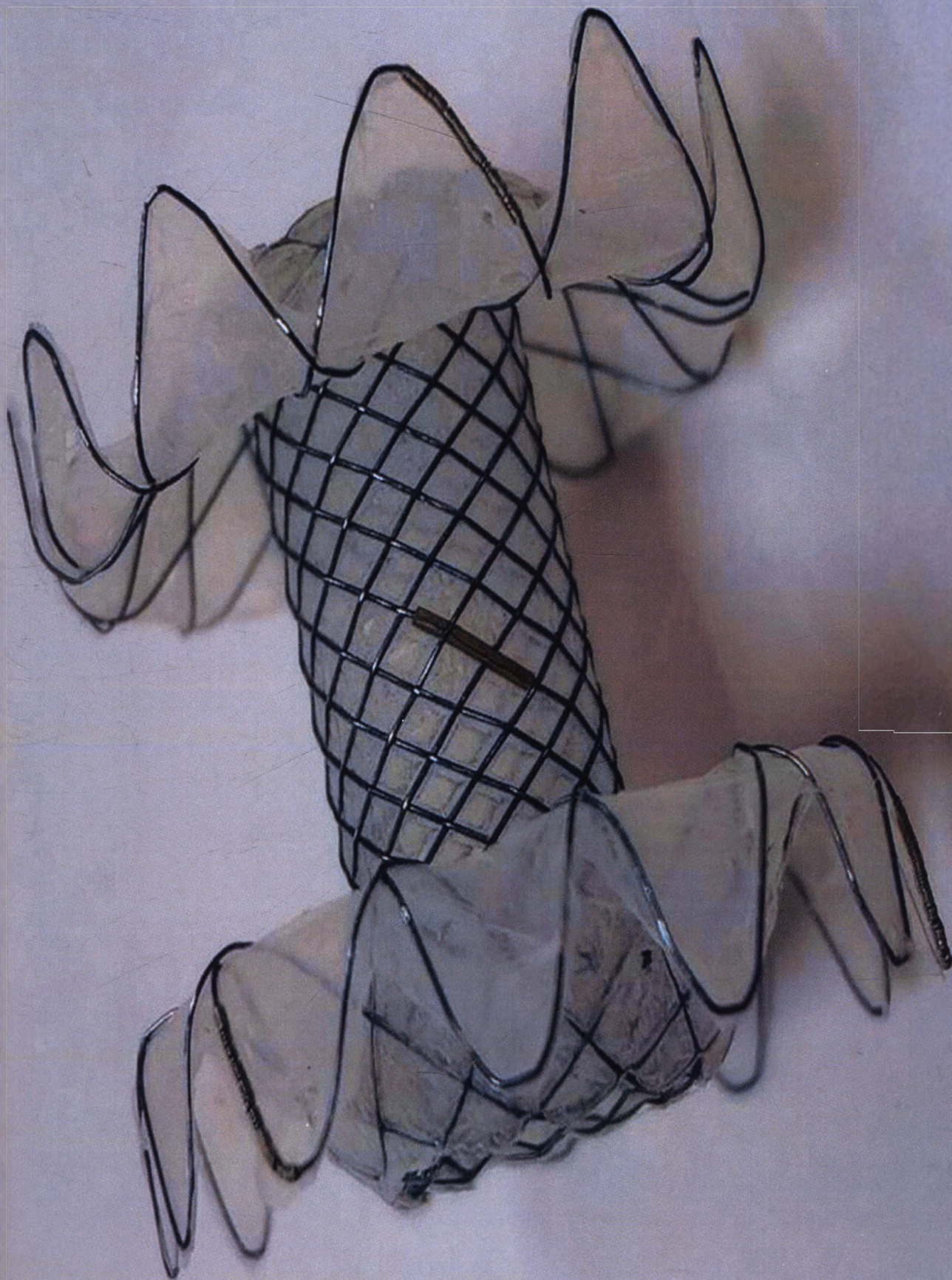
Стент в развернутом виде
