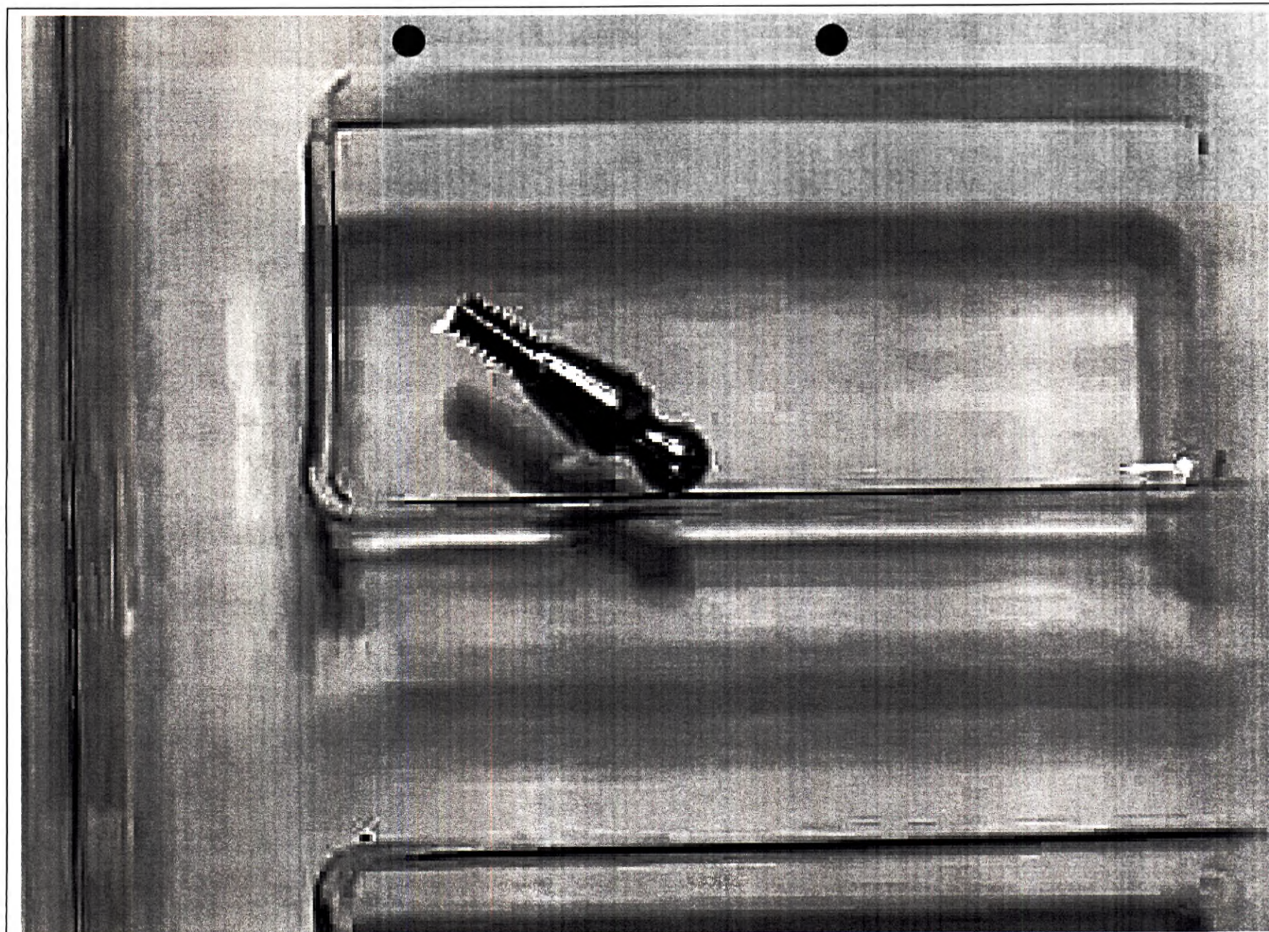
Абатмент Implantswiss Bone Level Mini O-Ring Abutment, Dimensions: Diameter - 2.9 mm, Gingival Height - 0.5 mm NON STERILE (артикул S-BMORA05)
