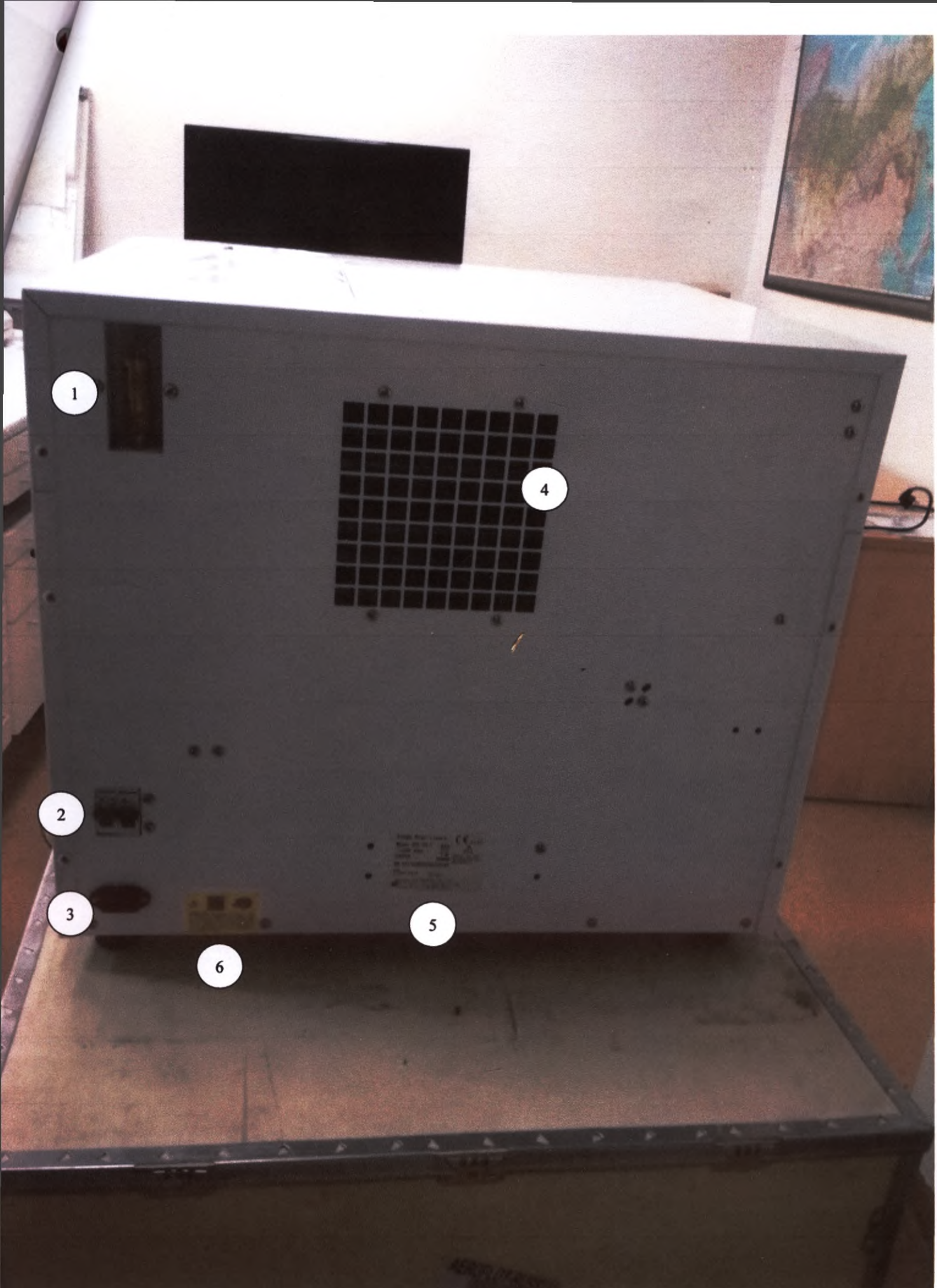
Рис. 18. Вариант исполнения STE-29-T, вид сзади. (Идентично для STE-29-T, STE-45-T). Клапан воздушного предохранителя (1); Автоматический электропредохранитель (2); Разъем для кабеля питания (3). Вентиляционное отверстие (4). Заводская маркировка (5). Место для заземления (6).
