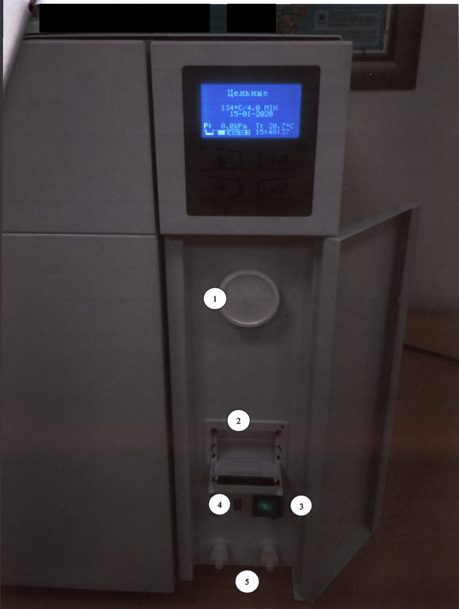
Рис. 16. Фильтр воздушный бактерицидный (1), Встроенный принтер (2), Кнопка Вкл/Выкл питания (3), USB-порт (4), Разъемы для слива дистиллированной воды (справа), и отработанной воды (слева), (5). Идентично для вариантов исполнений STE-29-T, STE-29-T.
