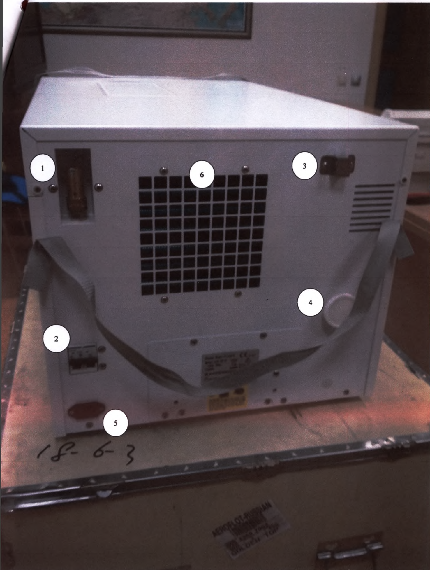
Рис. 3. Вариант исполнения STE-29-D вид сзади. (Идентично для STE-8-D, STE-18-D, STE-23-D, STE-29-D). Клапан воздушного предохранителя (1); Рычаг автоматического электропредохранителя (2); Отверстие для выхода пара из бака отработанной воды (3); Фильтр воздушный бактерицидный (4); Разъем для кабеля питания (5). Вентиляционное отверстие (6).
