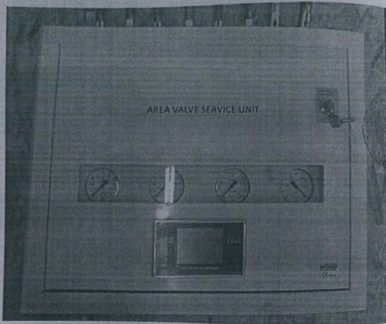
ФОТО 103. Блок контроля SZKG-4 (AREA VALVE SERVICE UNIT «SZKG»)
