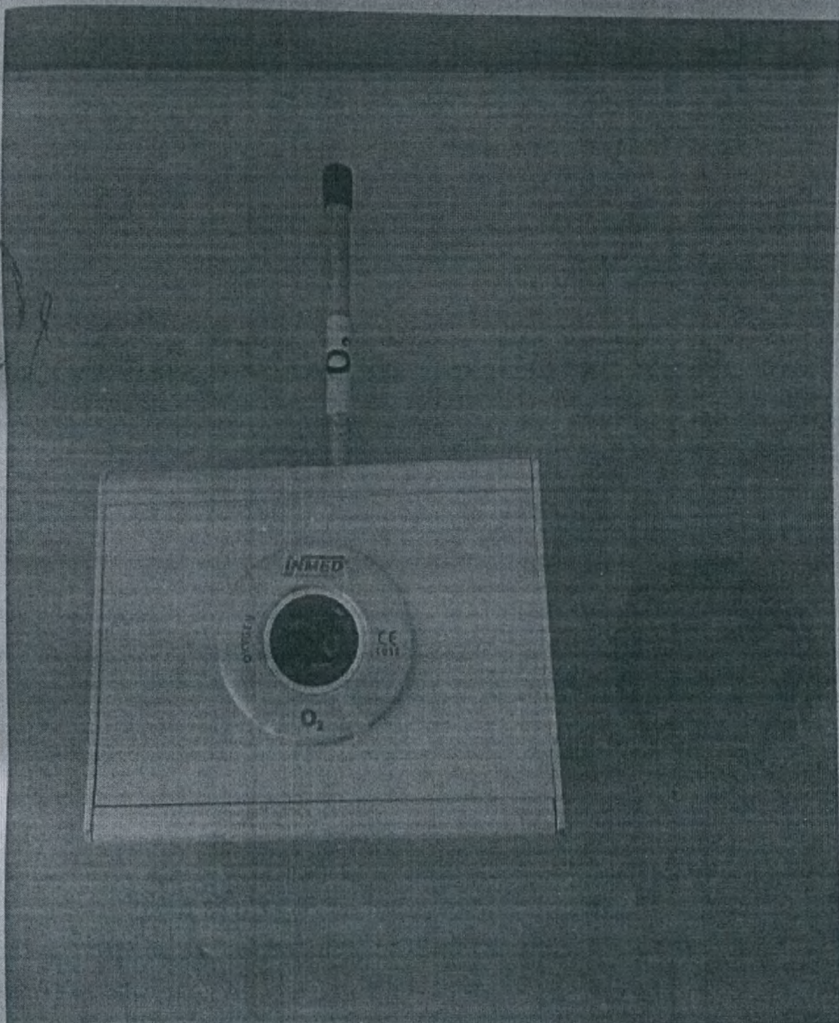
ФОТО 98. Газовая панель TPG (MEDICAL GAS CONSUMPTION BOARD) вариант исполнения TPG-N (вид спереди)
