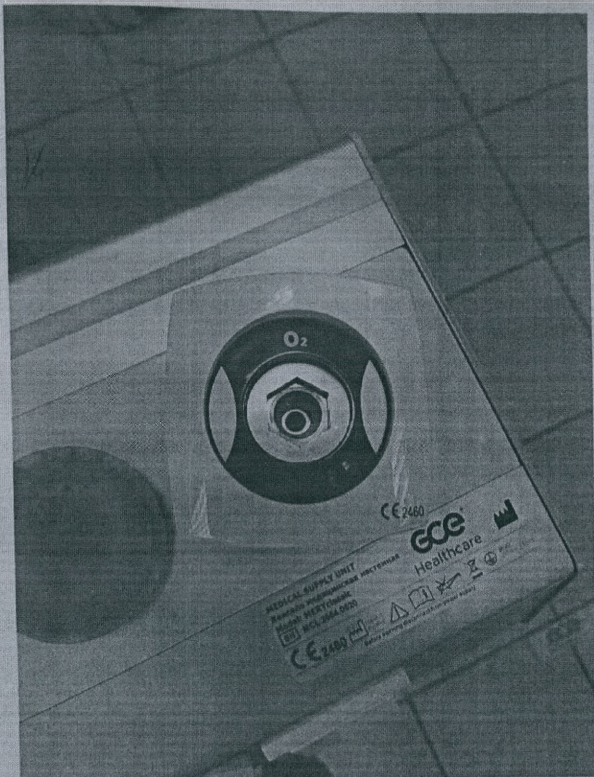
ФОТО 48. Разъем стандарта (gas outlet) BS 5682
