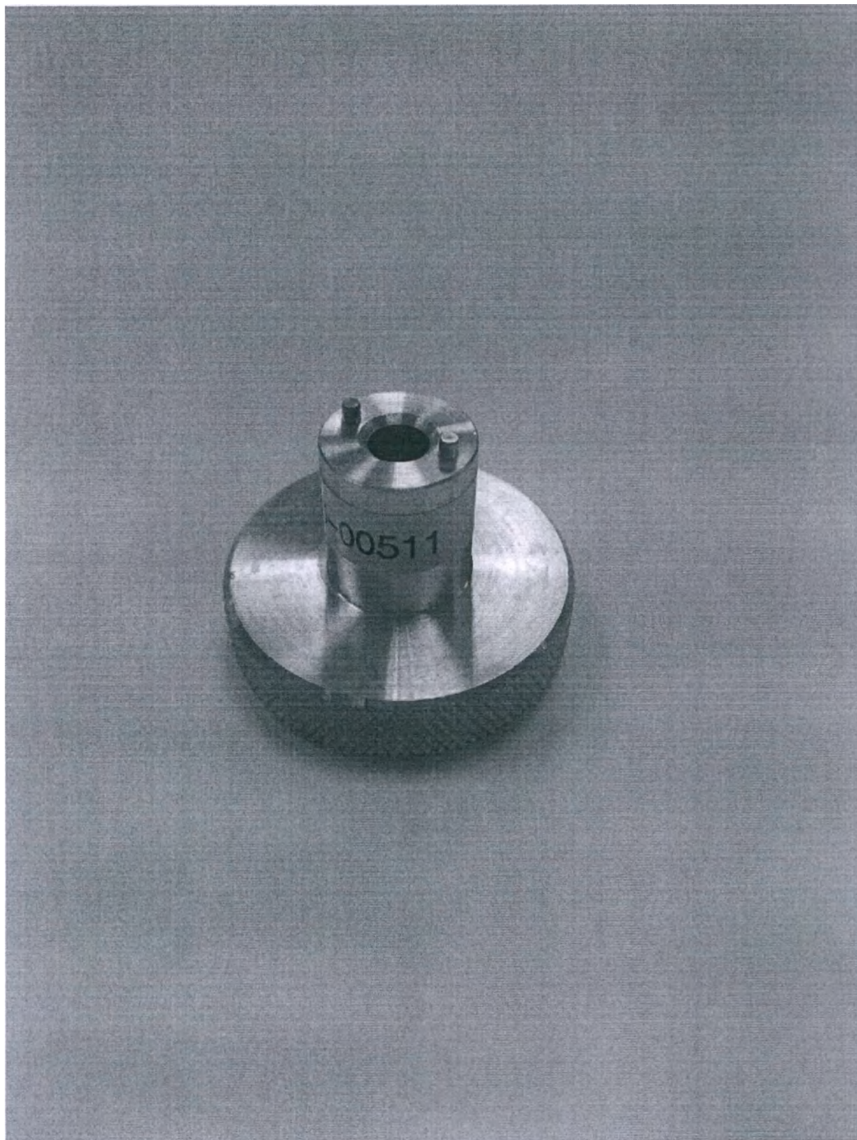
Фото №12. Ключ монтажный для выходного штуцера Zen-O™.
