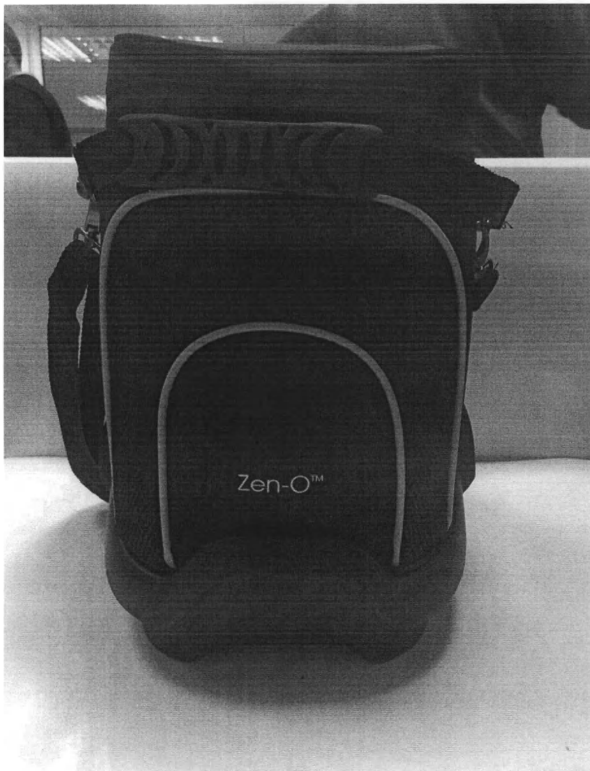
Фото №1. Концентратор Zen-O ™ в сумке-переноске Zen-O ™ . Вид спереди.
