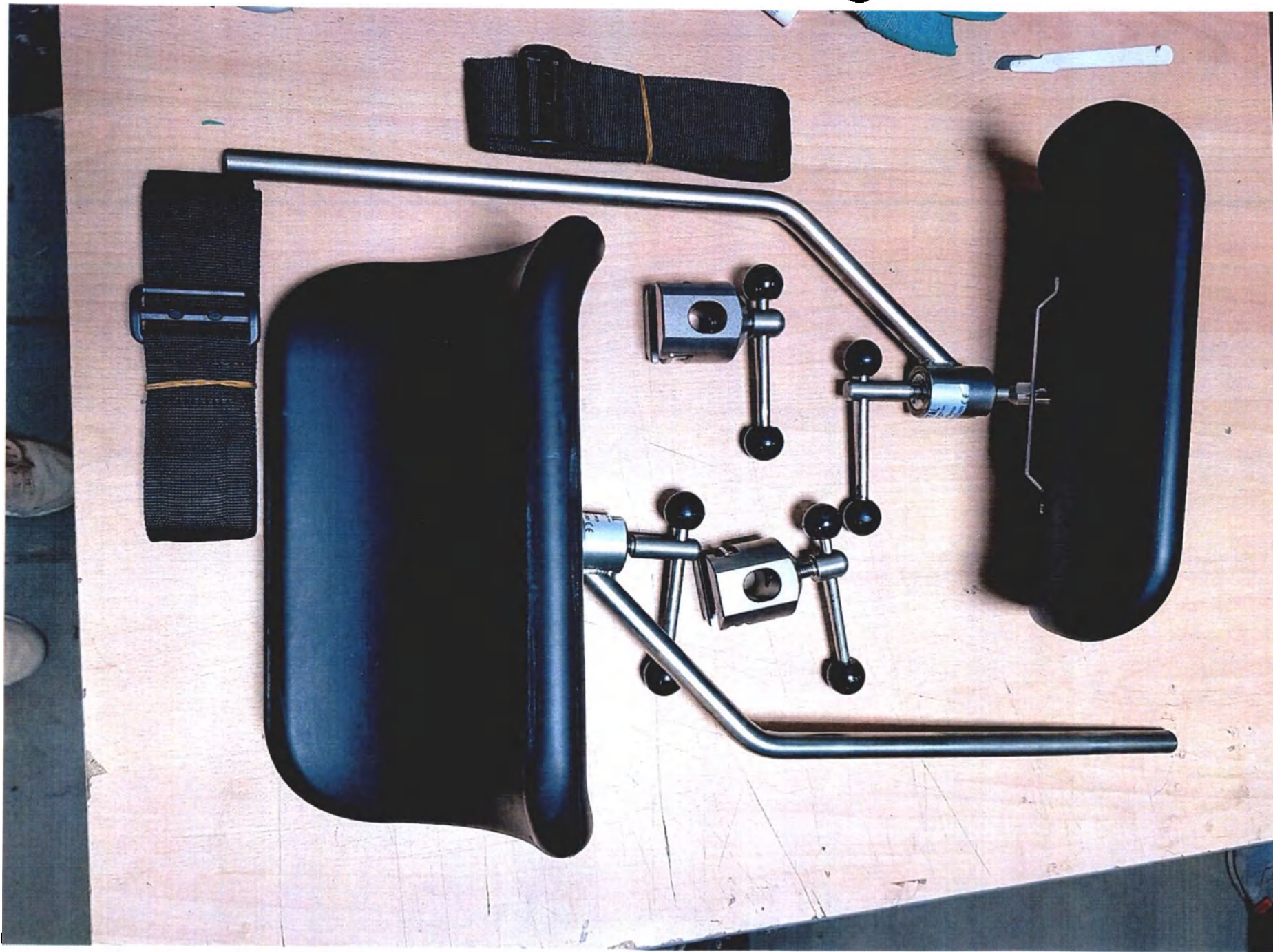
Опоры боковые
