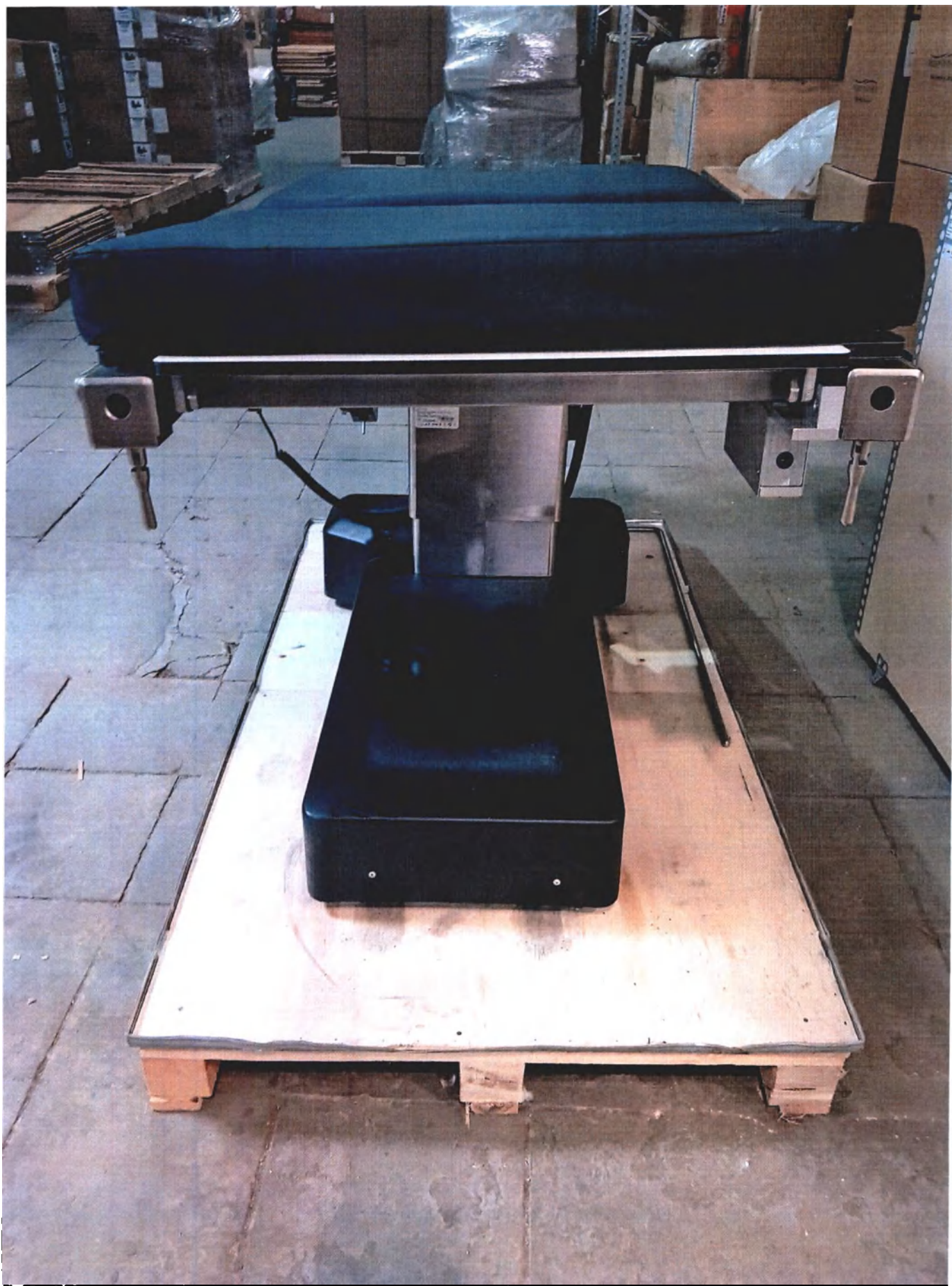
Стол операционный электрогидравлический-бариатрический ОТ80.15 в составе: секция спинная; секция тазовая; секции ножные, матрасы спинной секции, матрас тазовой секции, матрасы ножных секций, основание Т-образное из нержавеющей стали
