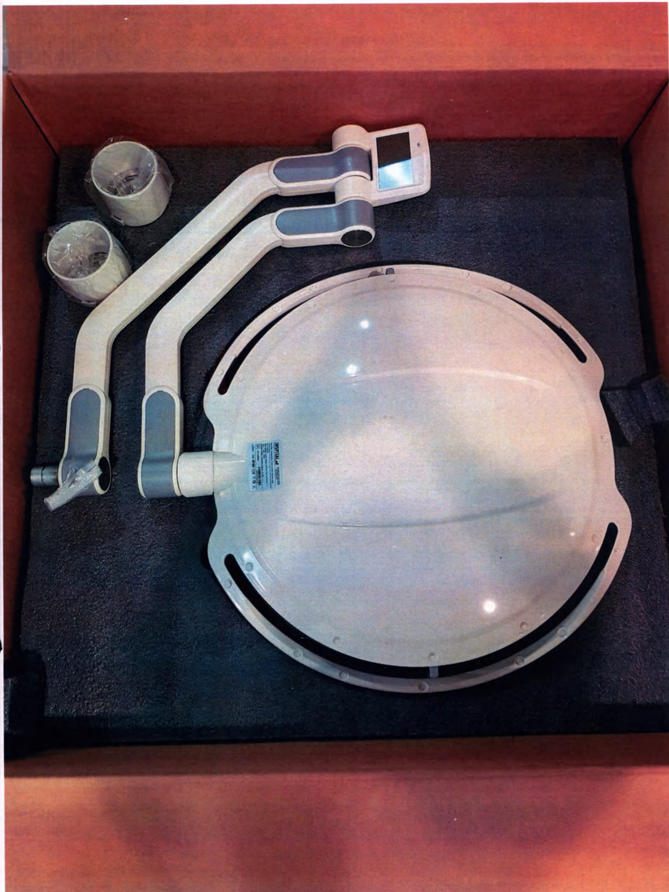
Светильник операционный бестеневой потолочный двухкупольный с монитором на рычаге, модель 20.53, в составе: купол светильника со светодиодными лампами; панель управления; рычаги серповидные (вид сзади).
