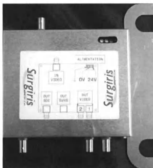
Блок управления камерой
