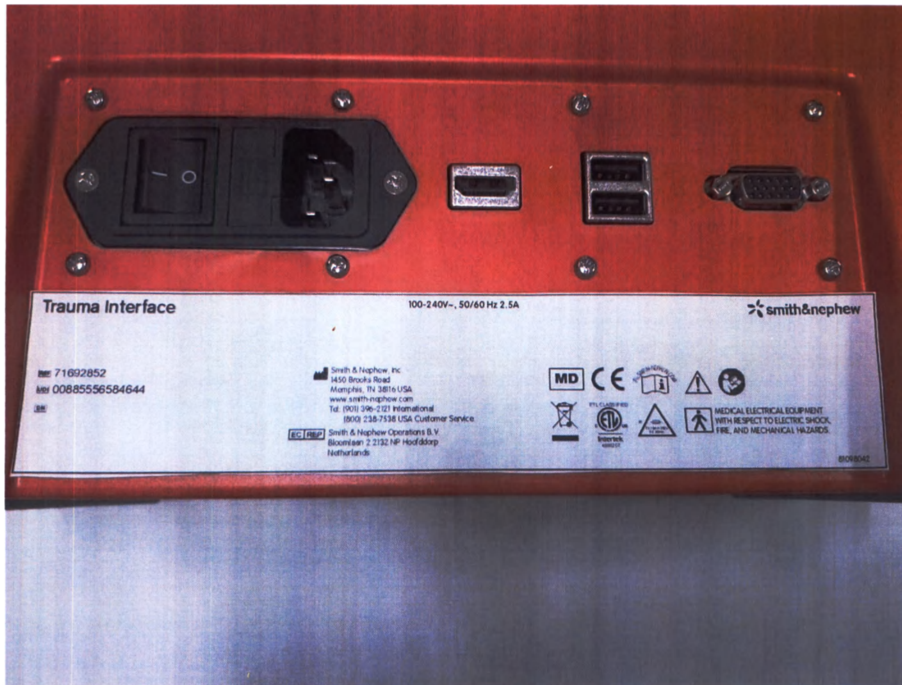
Рис. 6. Интерфейс TRIGEN SURESHOT, вид сзади, проект обновленной маркировки
