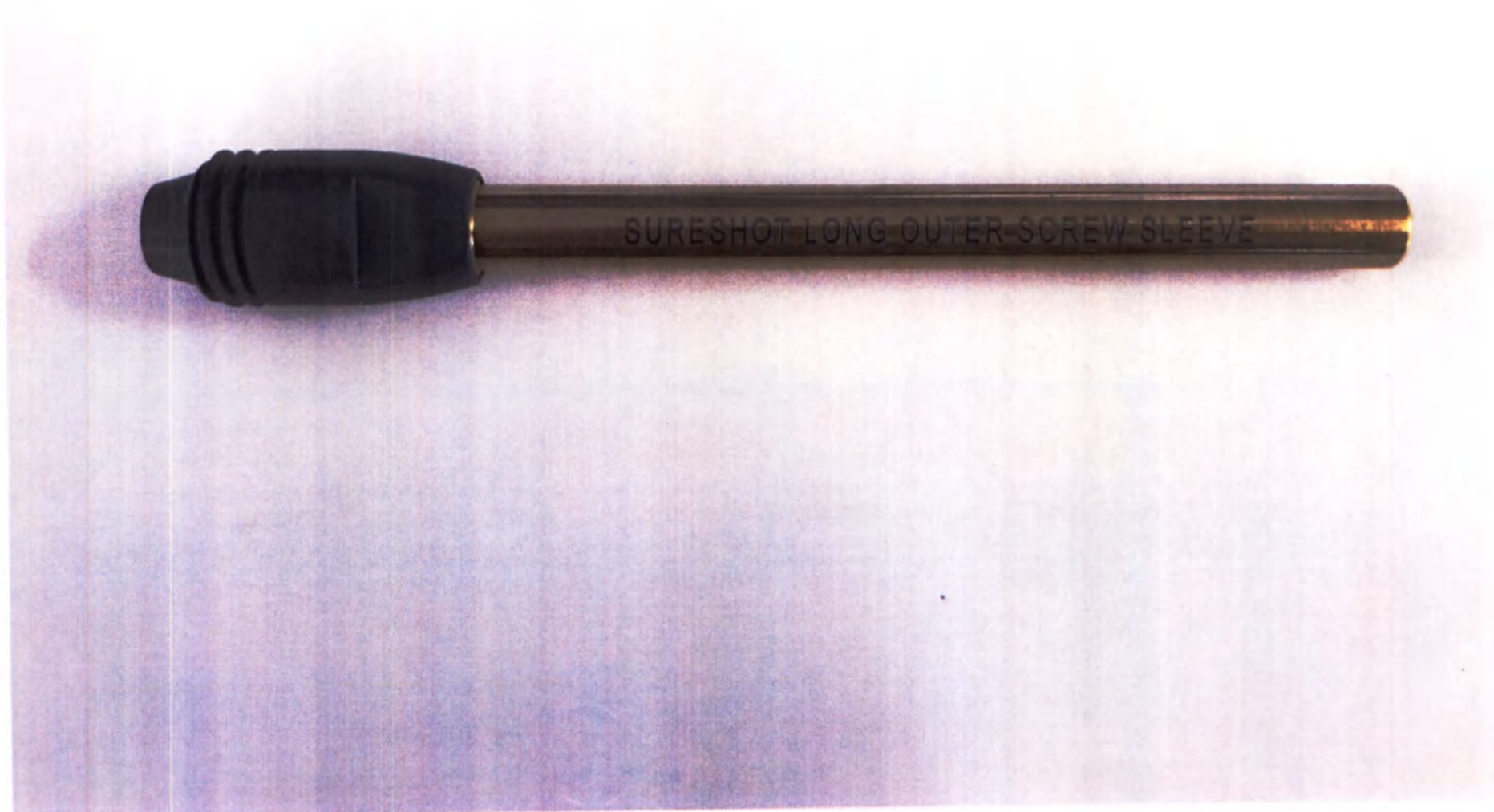
Рис. 13. Втулки SURESHOT: Втулка для винта SURESHOT, длинная
