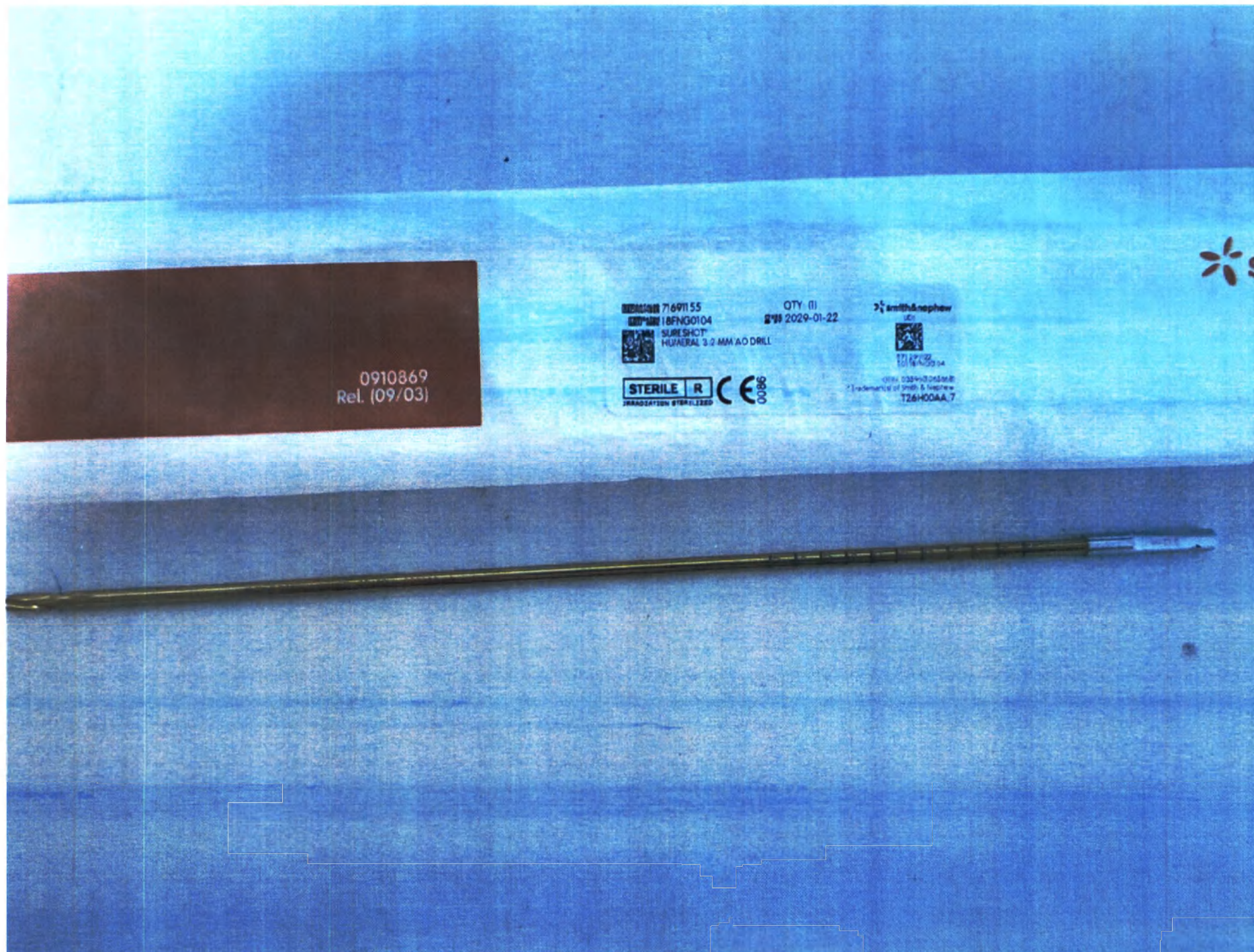
Рис. 38. Сверла SURESHOT (стартовый комплект): Сверло SURESHOT HUMERAL, хвостовик типа AO
