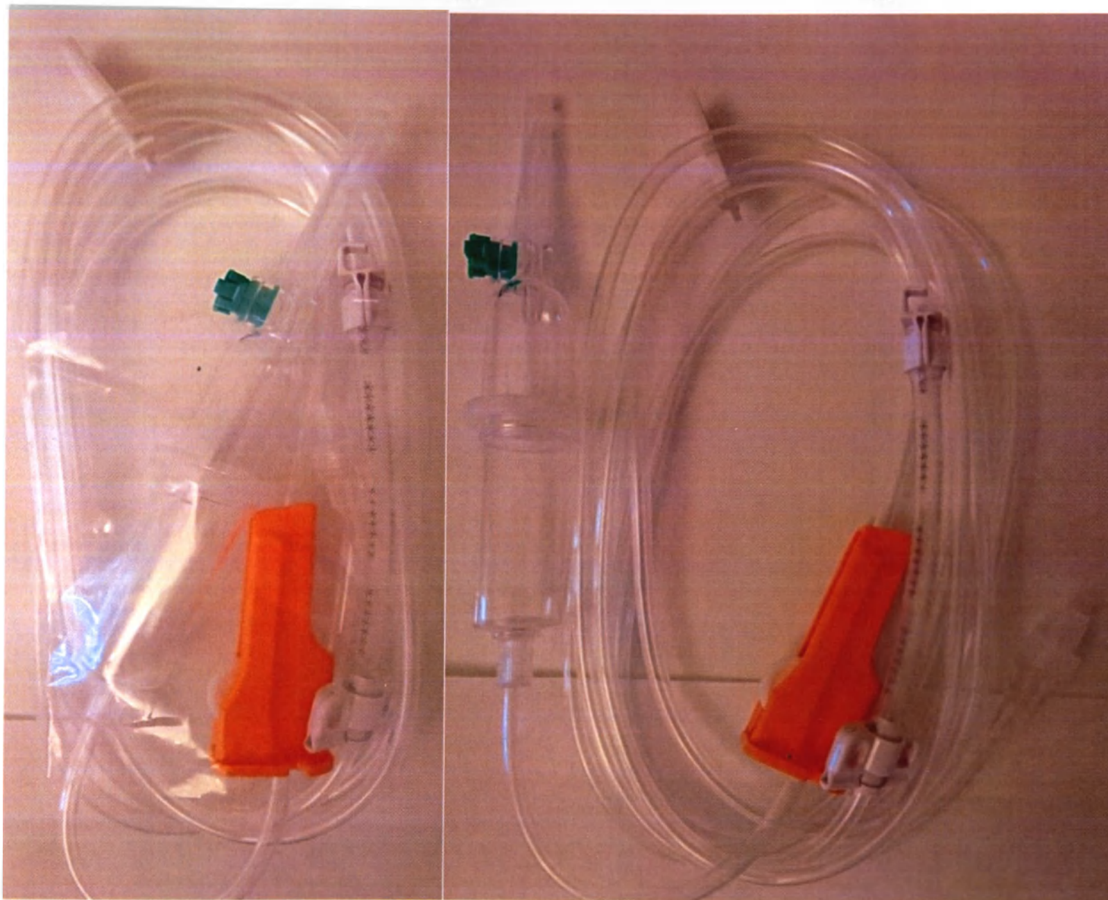
Рисунок 8 – «Магистраль Инфузомат® Спэйс (Infusomat® Space) для использования с совместимыми насосами и гравитационного введения, инфузионная: 8250731SP»: слева - с фиксирующей лентой из полиэтилена (для дополнительной сохранности в упаковке), справа - медицинское изделие без фиксирующей ленты
