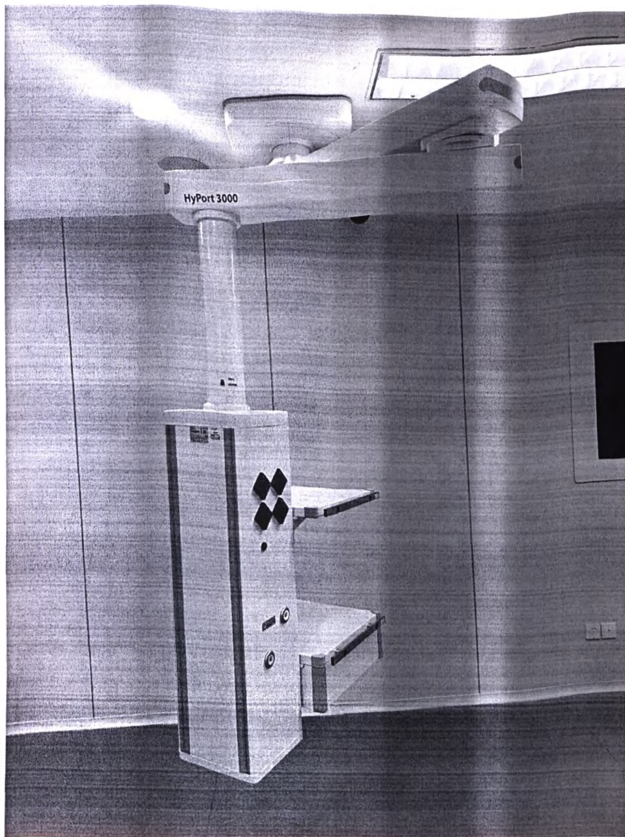
Консоль медицинская HyPort для подвода медицинских газов и подключения аппаратуры, с принадлежностями, вариант исполнения HyPort 3000
