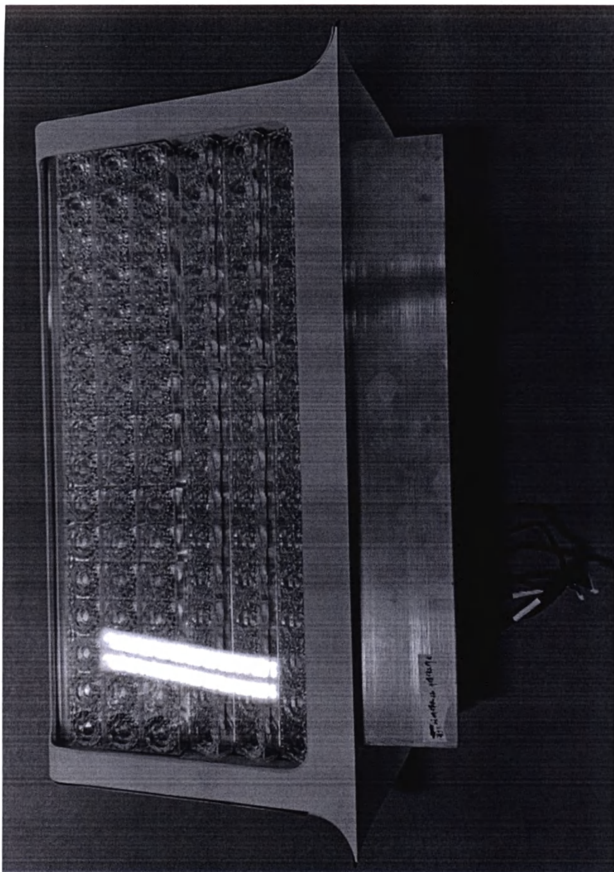
Светильник интеллектуальный встраиваемый с модулем управления
