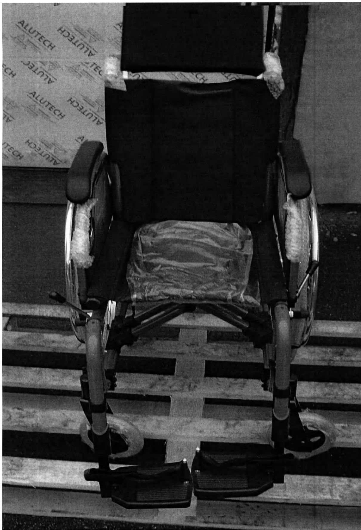
Коляски механические Invamedica Серия N Line, модель N Line 17 (Ширина сиденья 355 мм, 380 мм, 405 мм, 430 мм, 455 мм, 480 мм, 505 мм, 530 мм, 555 мм)
