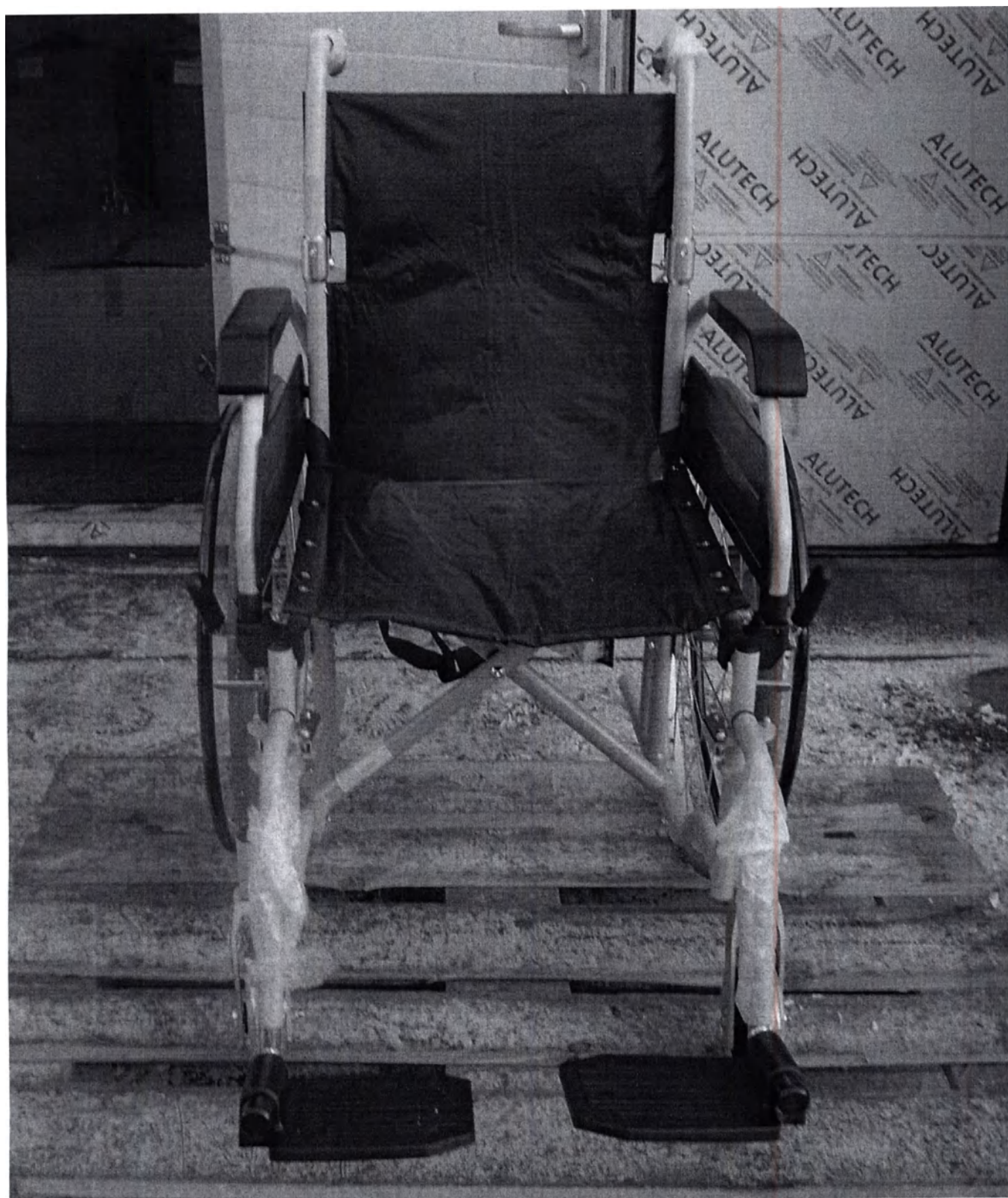
Коляски механические Invamedica Серия N Line, модель N Line 25 (Ширина сиденья: 380 мм, 405 мм, 430 мм, 455 мм, 480 мм, 505 мм, 530 мм, 555 мм)
