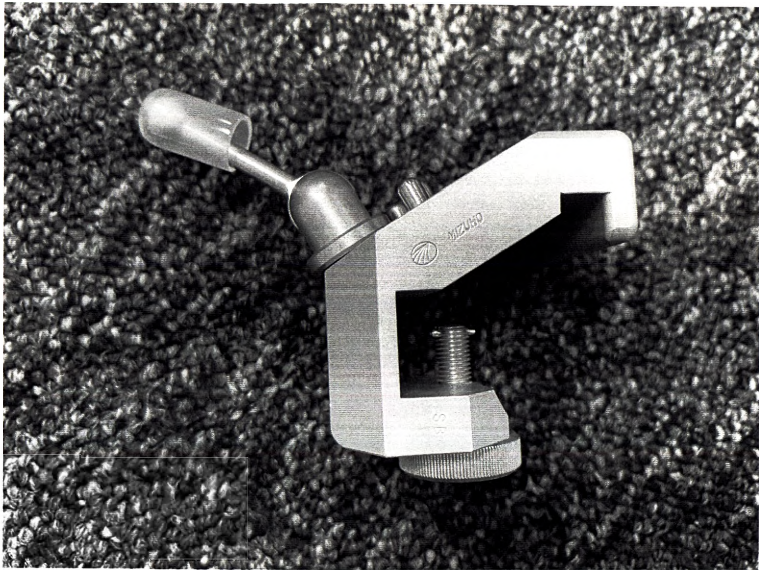
Фото 8. Регулятор скольжения для ретрактора
