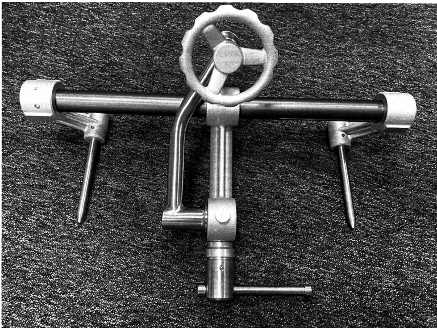
● Фото 13. Крепление к столу
