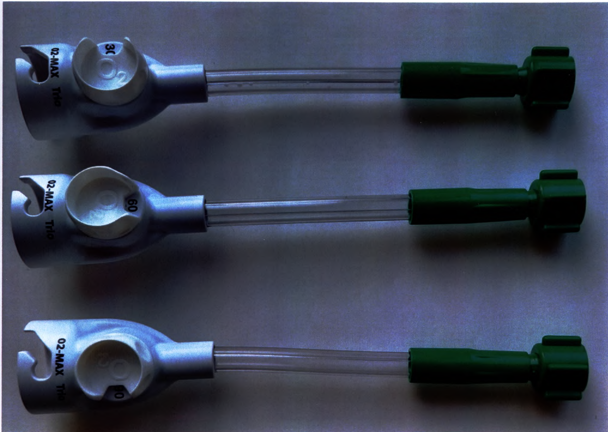
Трубка кислородная со ступенчатым регулятором FiO 2
