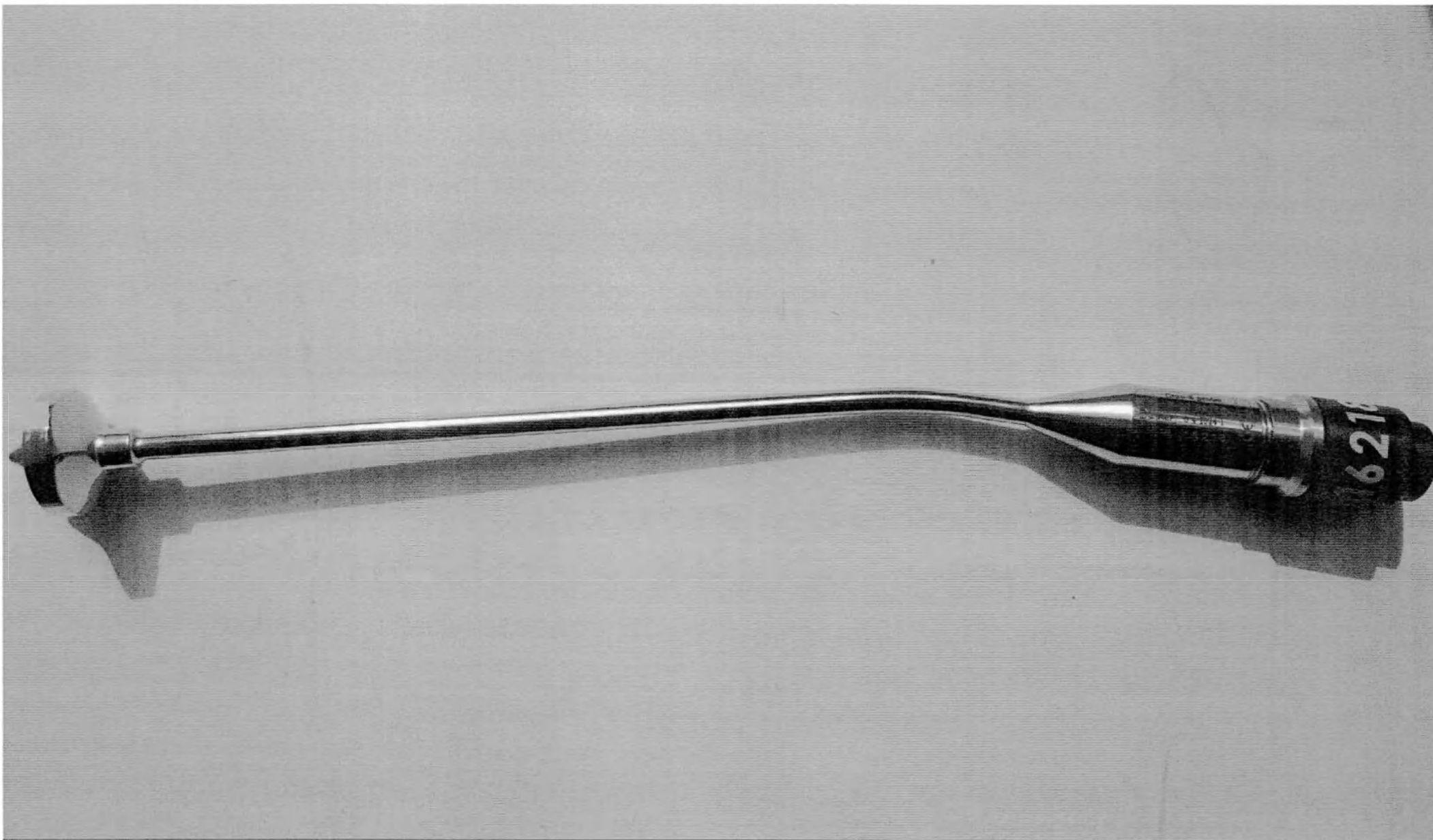
Криозонд контактный многоразовый типа G-10/24/RF, номер по каталогу: 0 4 1024 1 (в составе Аппаратов криохирургических «Cryo-S Painless» и «Cryo-S Painless»)
