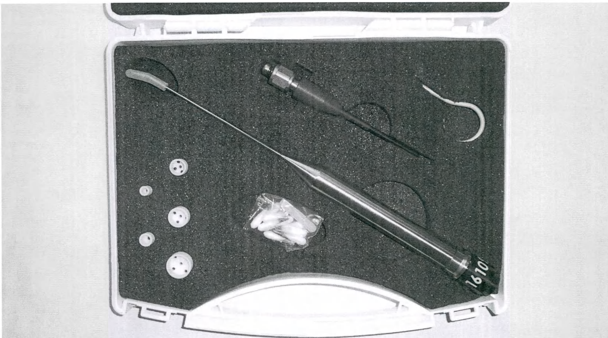
Криозонд распылительный многоразовый типа SG-10, номер по каталогу: 0 4 0000 1, в составе: Криозонд распылительный многоразовый типа SG-10, номер по каталогу: 0 4 0000 1 – 1 шт.; Ограничитель области заморозания гинекологический – 5 шт.; Адаптер для разблокировки распылительной насадки – 1 шт.; Инструмент для подготовки ватных палочек – 1 шт.; Палочки ватные нестерильные – 10 шт.; Колпачок защитный распыляющего сопла – 2 шт.; Бокс пластиковый – 1 шт. (в составе Аппаратов криохирургических «Cryo-S Painless» и «Cryo-S Painless»)
