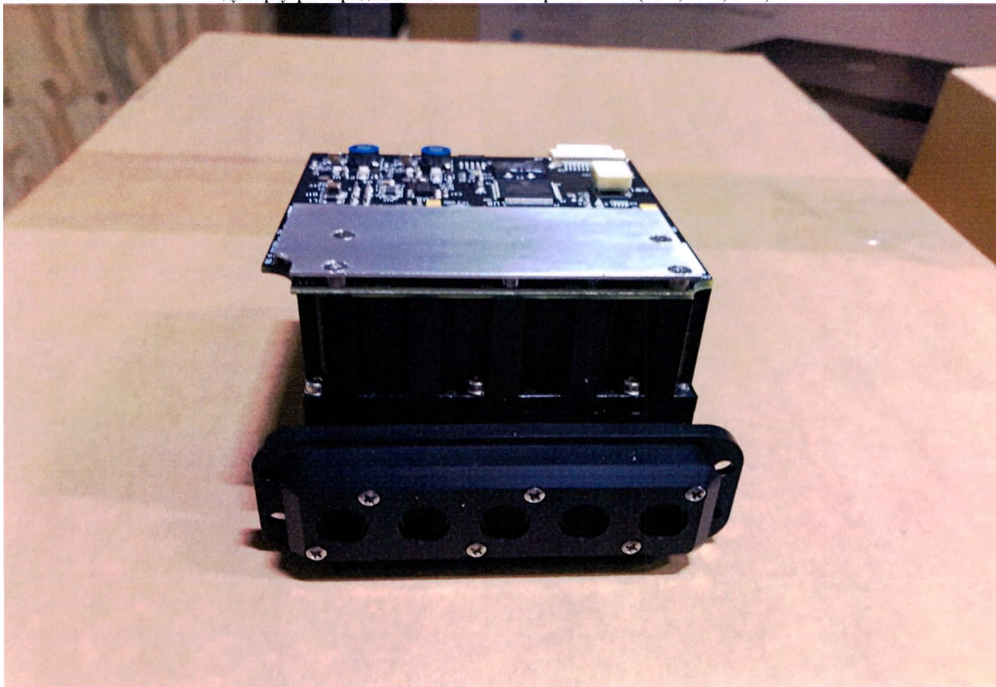
Модуль флуориметра для монтажа в анализатор PANTHER (ROX, FAM, HEX)
