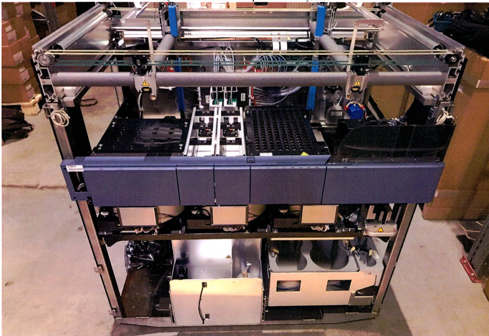
Модуль основной анализатора PANTHER System
