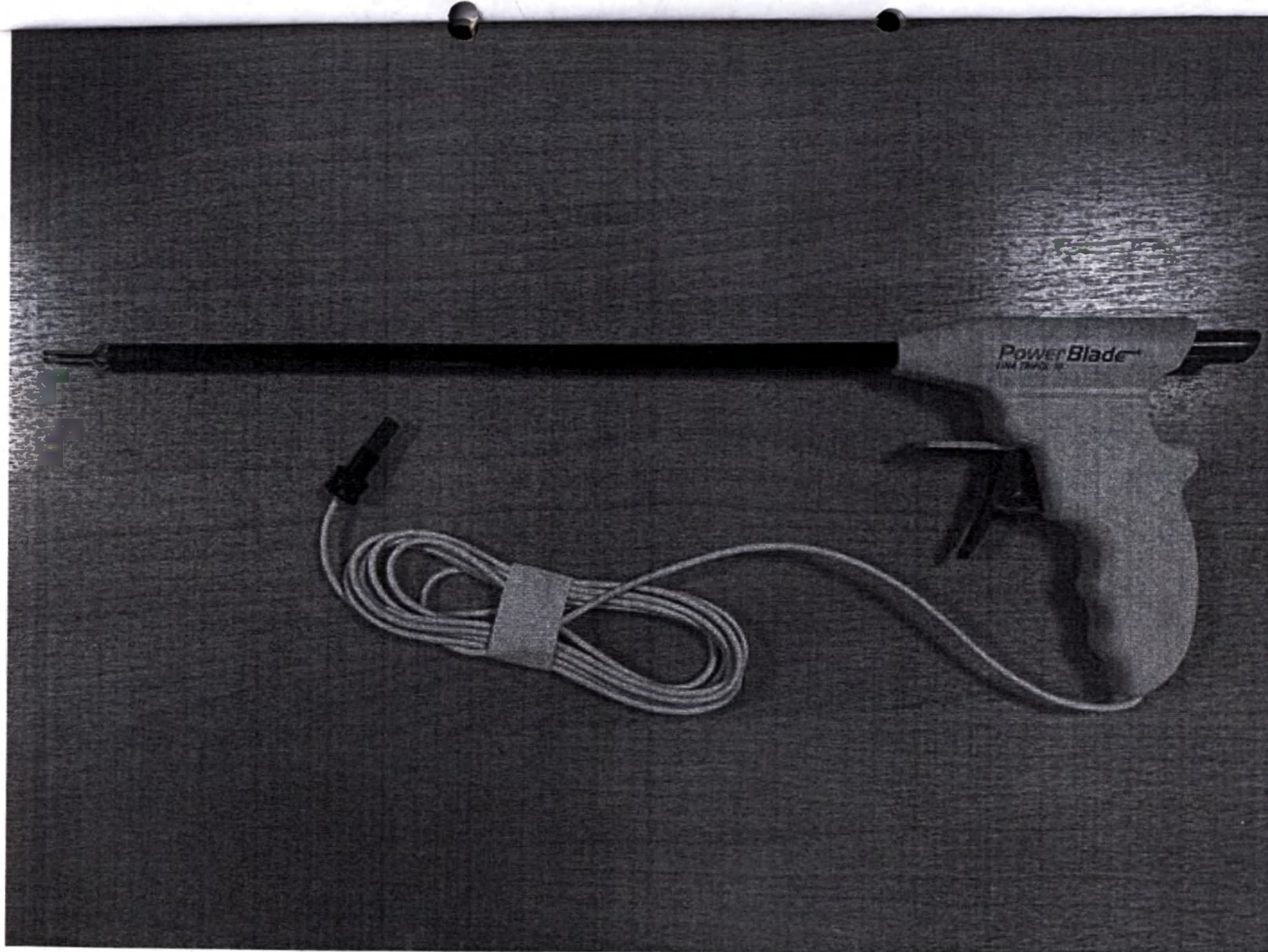
Щипцы биполярные для резки и коагуляции LINA PowerBlade 5010-E-RU
