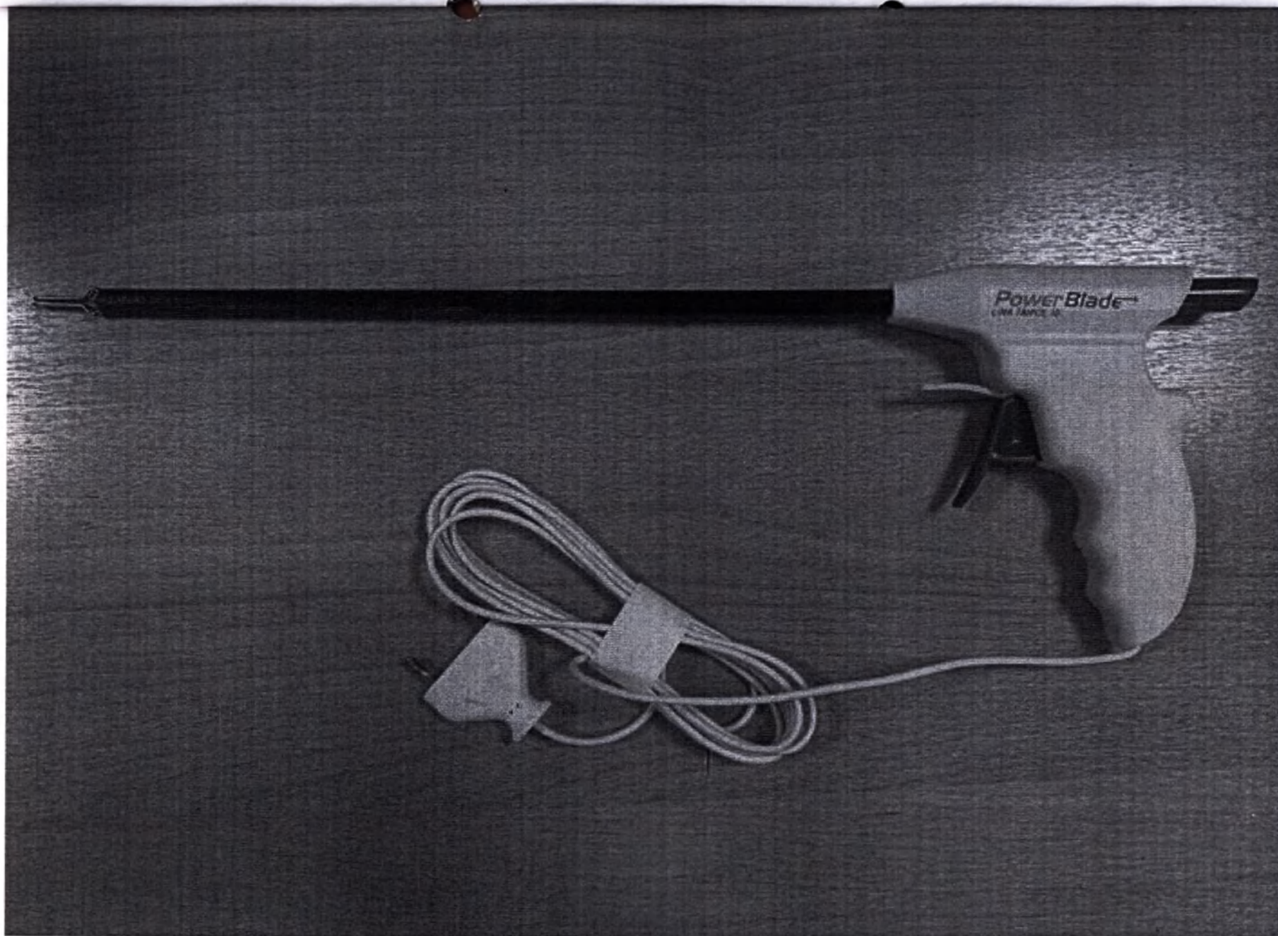
Щипцы биполярные для резки и коагуляции LINA PowerBlade 5010-Y-RU
