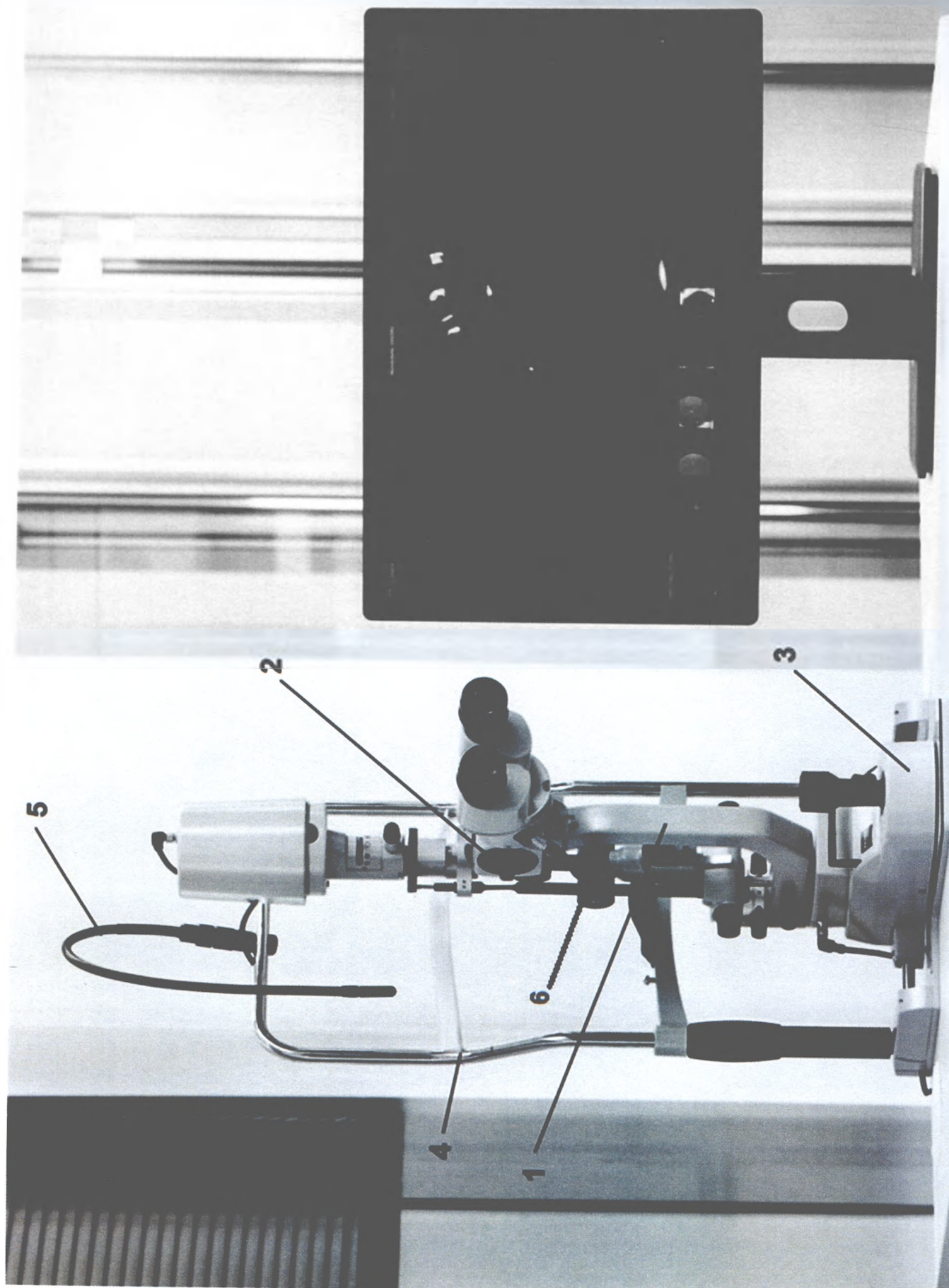
1. Лампа щелевая SL 220, 2. Стереомикроскоп с устройством смены увеличения (3- или 5-ступенчатым), бинокулярным тубусом (конвергентный или параллельный тубус) и окулярами 3. Основание прибора 4. Подголовник с опорой для подбородка 5. Внешняя фиксационная метка 6. Щелевой проектор
