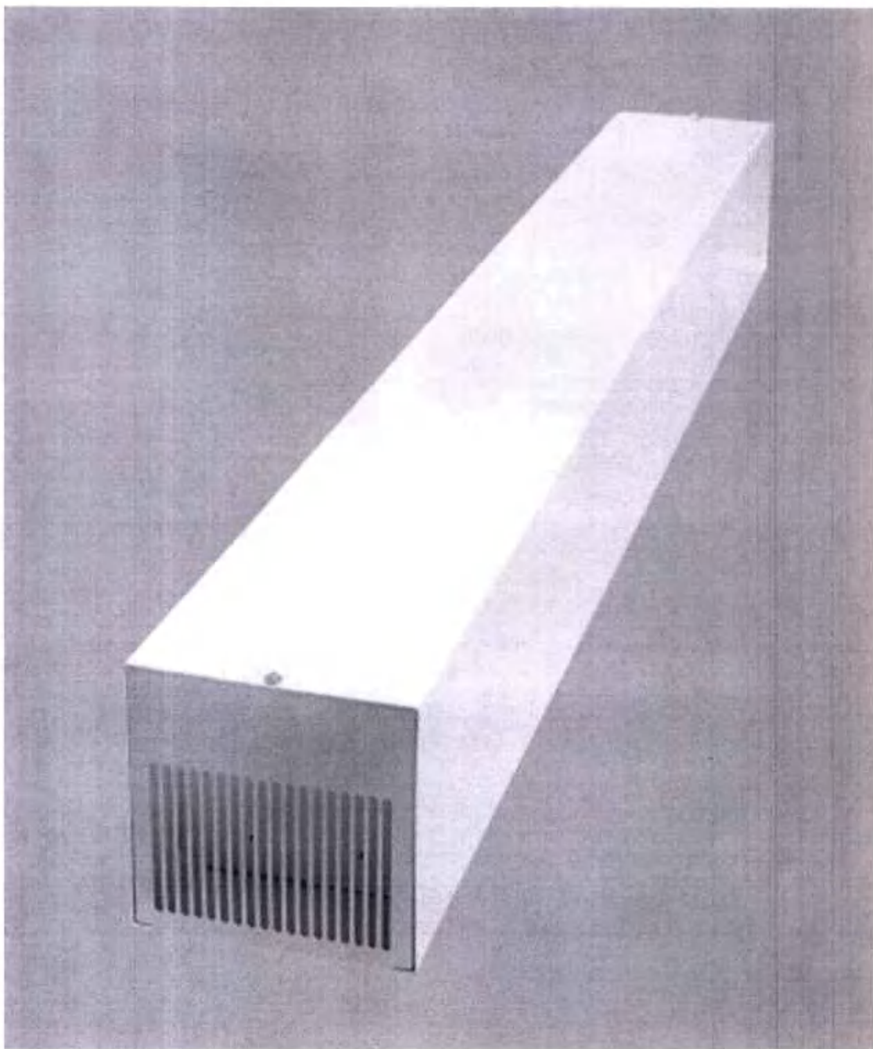
Рисунок 3 - Внешний вид моделей ОБРН01-1х30-112-00, ОБРН01-1х30-112-01, ОБРН01-1х30-112-11, ОБРН01-2х30-112-10, ОБРН01-2х30-112-00, ОБРН01-2х30-112-01, ОБРН01-2х30-112-11, ОБРН01-2х30-112-10
