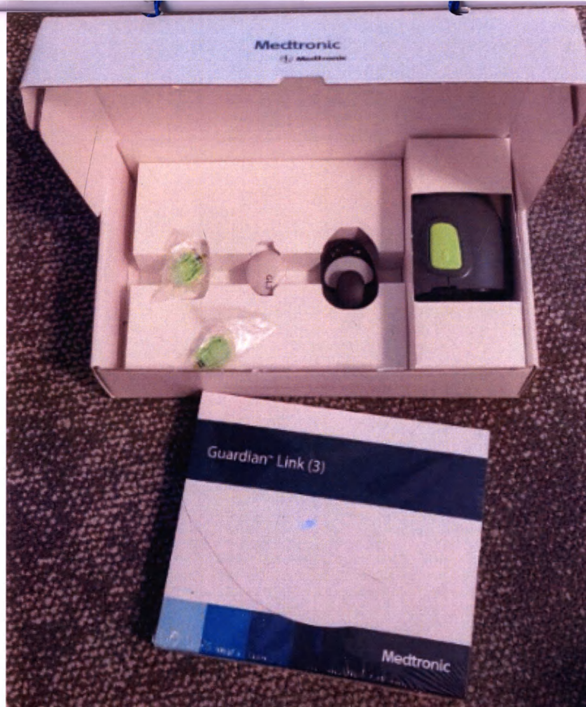
Набор трансмиттера Guardian Link (3), номер по каталогу MMT-7910W3 – комплект поставки
