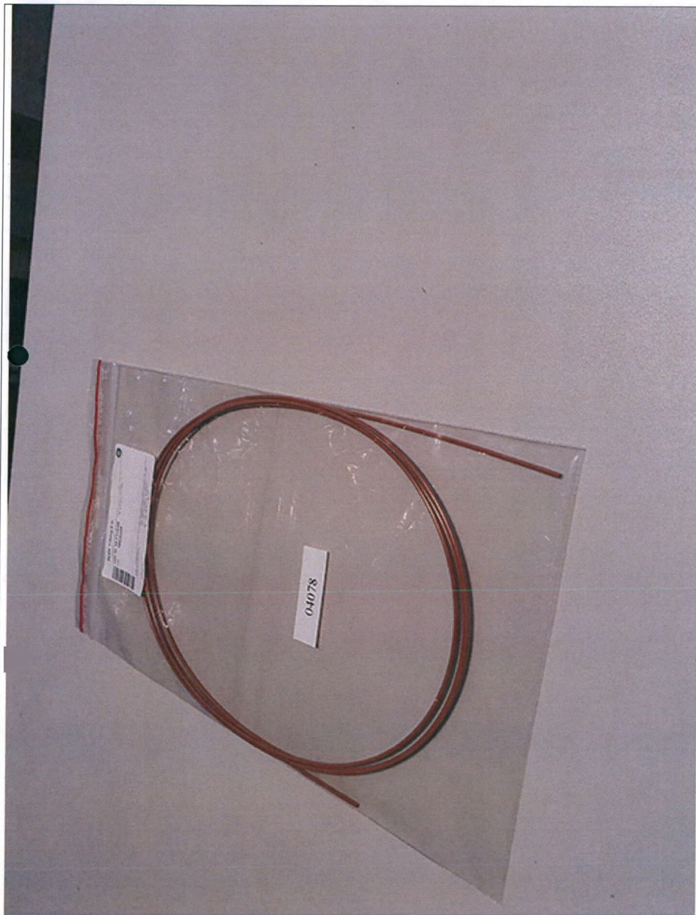
Внешний вид компонента медицинского «Анализатор иммунохемилюминесцентный автоматический «Люминит» (Luminite) с принадлежностями»: 15. Набор с трубками и инструментами: 15.10. Полиэфирэфиркетоновая трубка Ø 0,5X1,6 мм (2 м)
