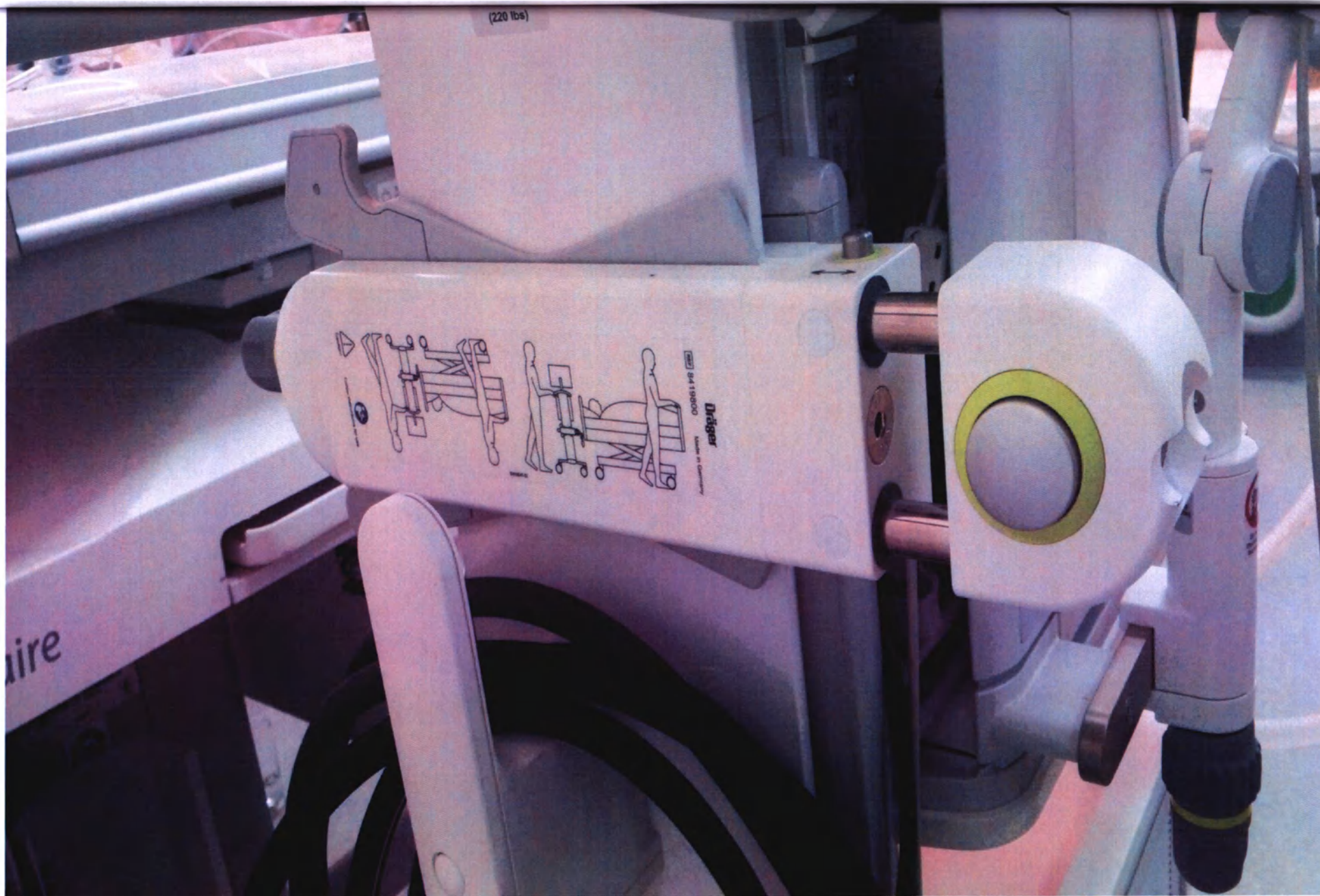
17. Замок для узла соединения с кроватью (сторона кровати).
