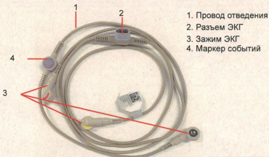
Рисунок 19 Кабель ЭКГ на 3 отведения
