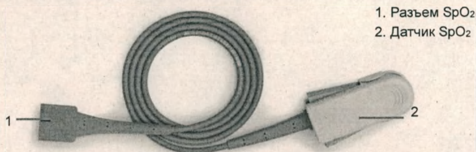
Рисунок 20 Датчик SpO 2
