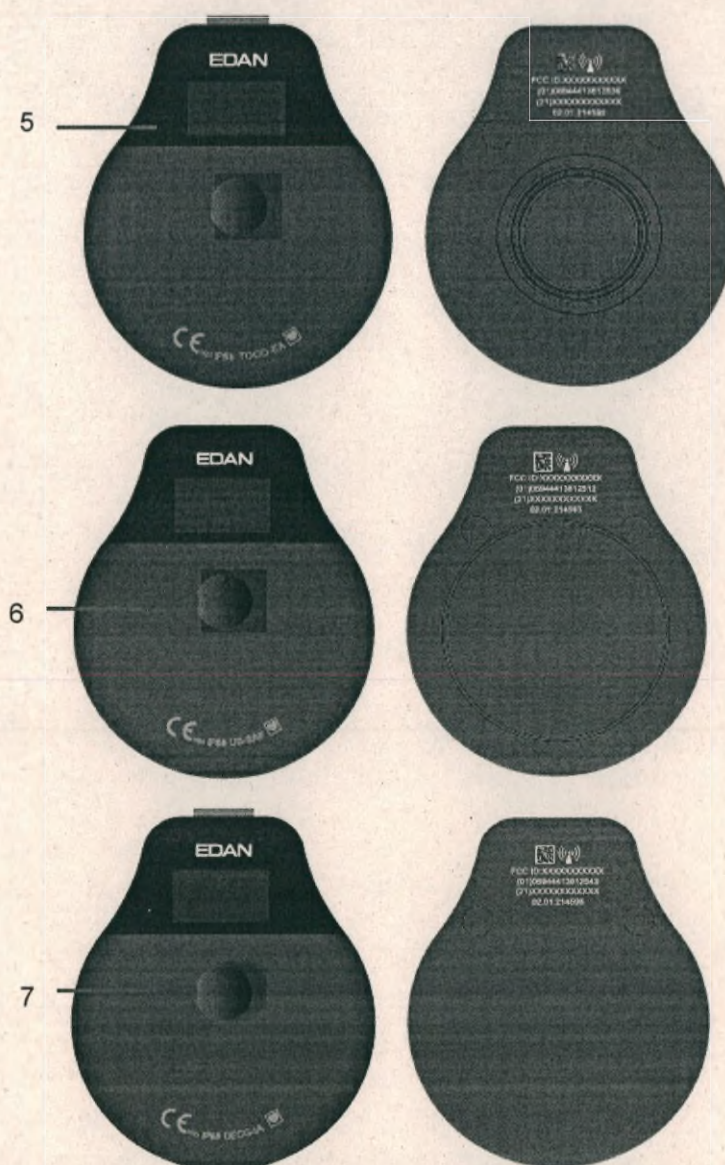
Рисунок 8 Беспроводные датчики
