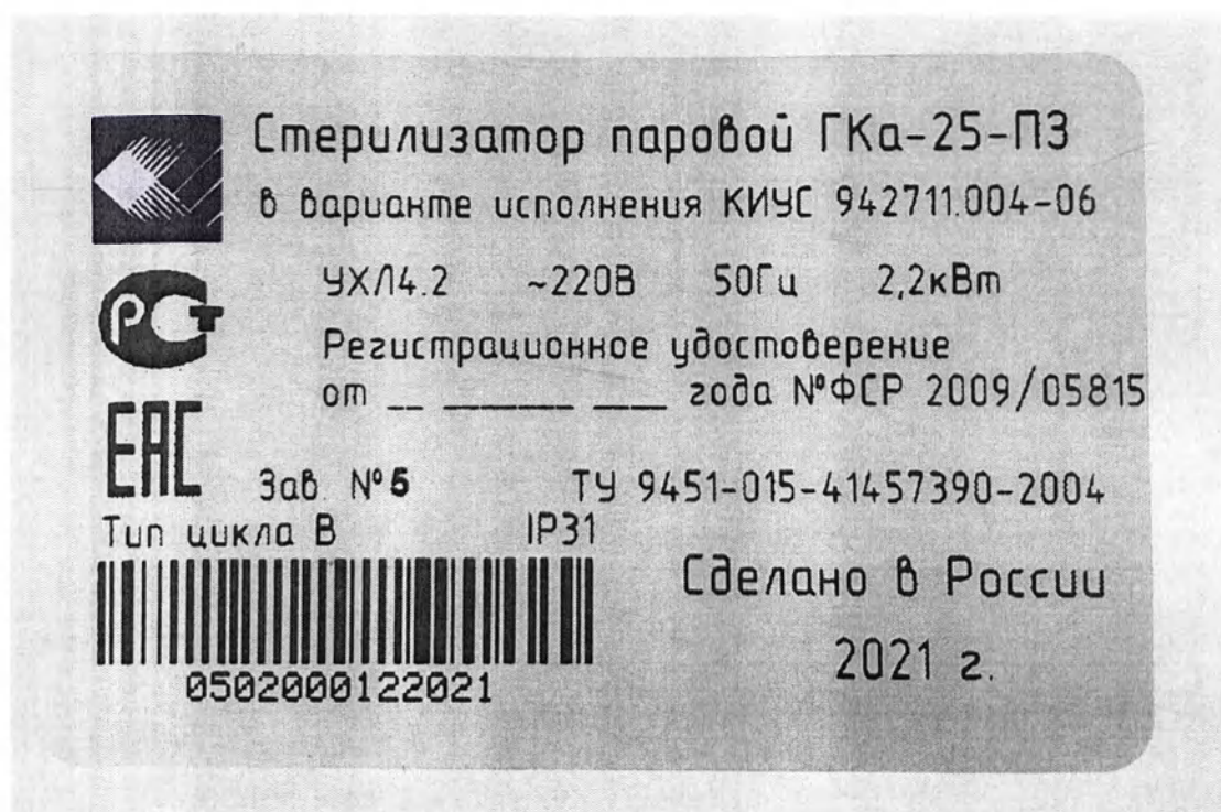
Фотографическое изображение 6. Стерилизатор паровой ГКа-25-ПЗ в варианте исполнения КИУС.942711.004-06
