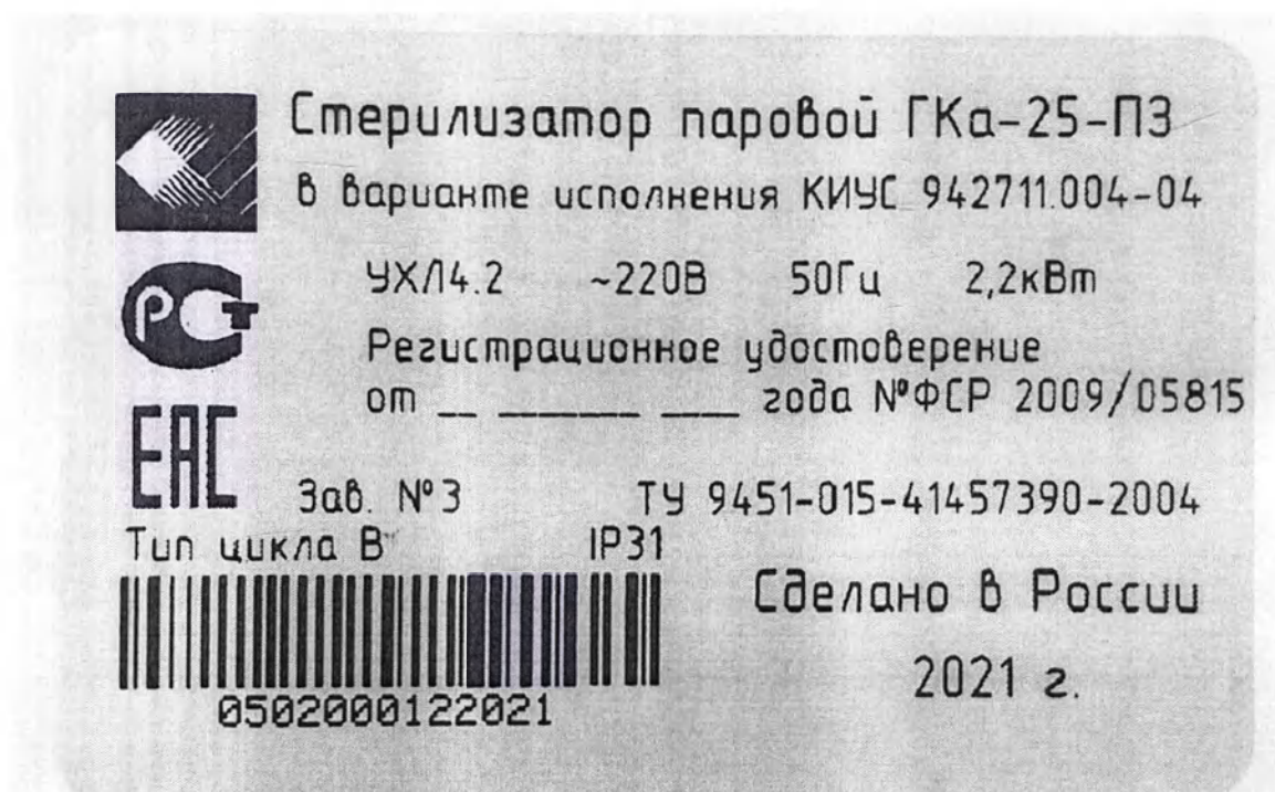
Фотографическое изображение 2. Стерилизатор паровой ГКа-25-ПЗ в варианте исполнения КИУС.942711.004-04 Маркировочная табличка
