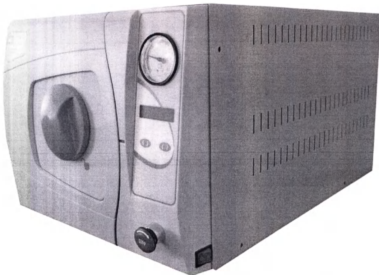
Фотографическое изображение 1. Стерилизатор паровой ГКа-25-ПЗ в варианте исполнения КИУС.942711.004-04
