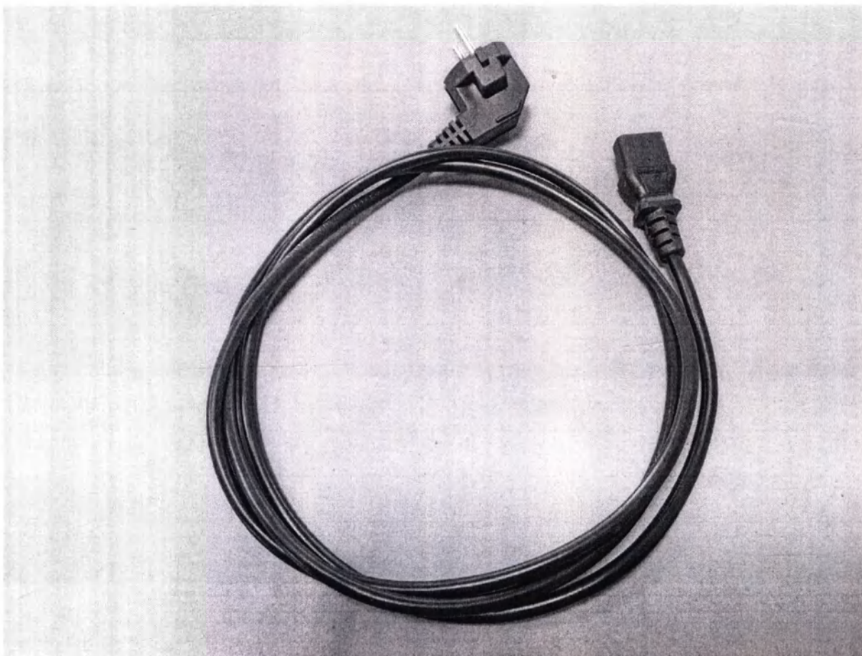
Фотографическое изображение 21. Евровилка с кабелем 10А 250В
