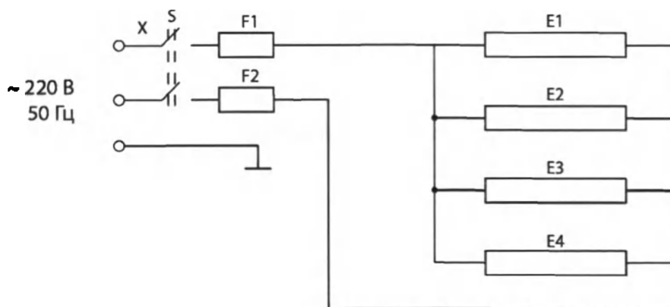
Рисунок 4. Схема принципиальная Негатоскопа общего назначения Нег-Н-РМ, исполнения 01СЛ (со светодиодными лампами):
