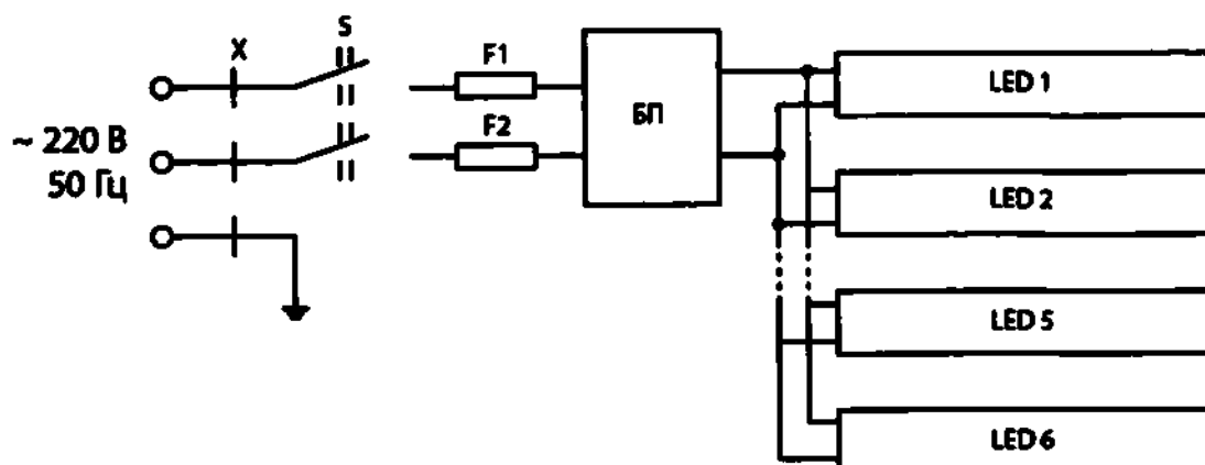
Рисунок 3. Схема принципиальная Негатоскопа общего назначения Нег-Н-РМ, исполнения 03С (со светодиодными линейками):
