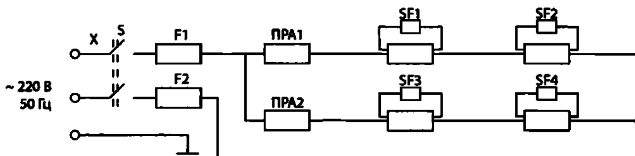
Рисунок 2. Схема принципиальная Негатоскопа общего назначения Нег-Н-РМ, исполнения 01 (люминесцентными с лампами):
