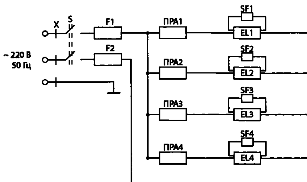
Рисунок 2. Схема принципиальная Негатоскопа общего назначения Нег-Н-РМ, исполнения 02 (с люминесцентными лампами):
