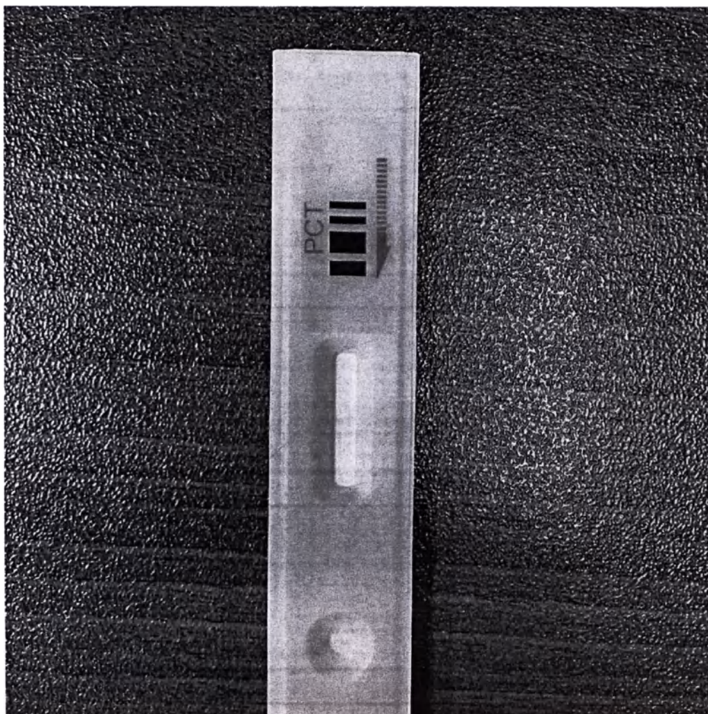
Тест-кассета для количественного определения прокальцитонина (PCT) иммунофлуоресцентным методом.
