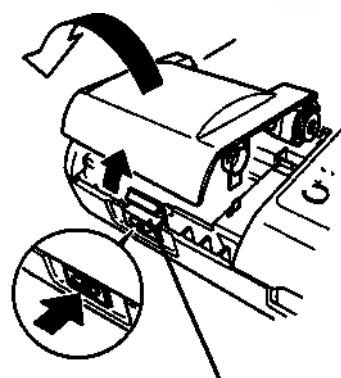
Кнопка открытия крышки самописца
