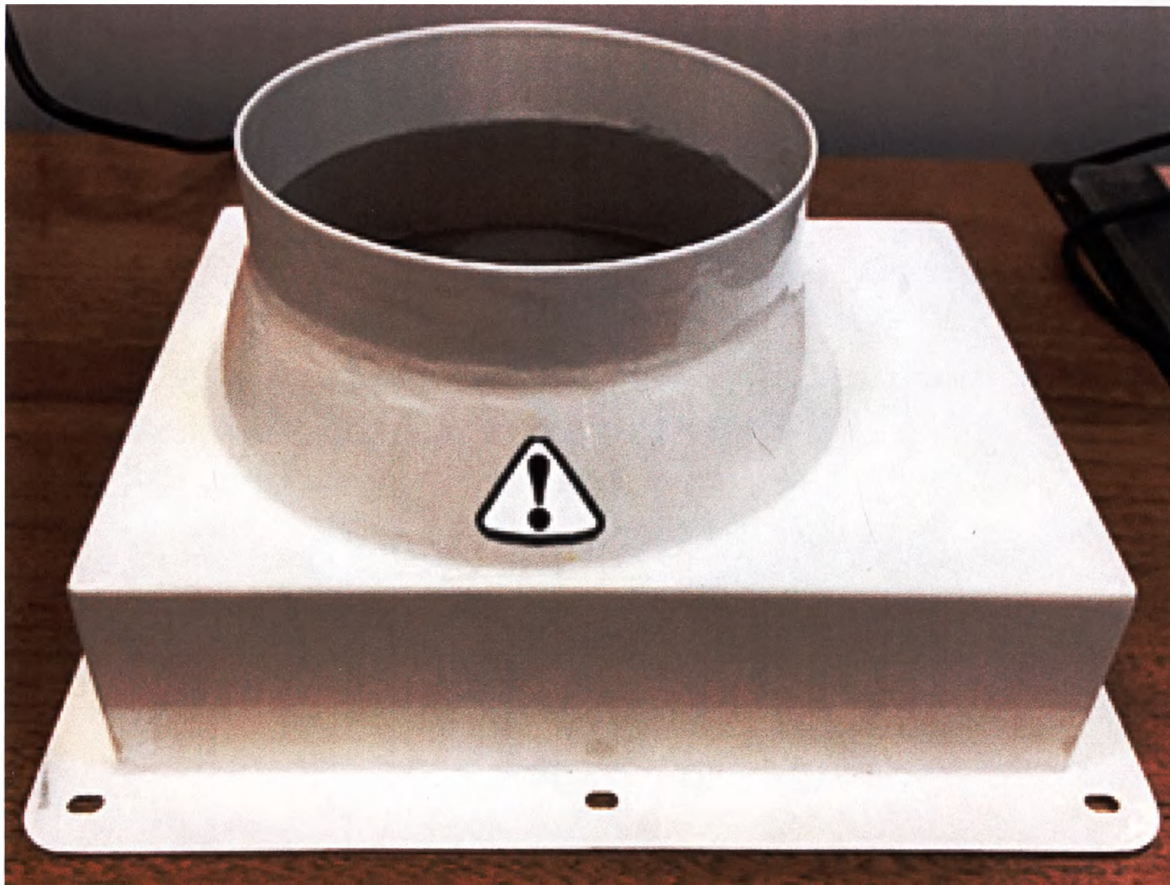
23. Внешний корпус вентиляционного выхода (Rear fan air guide weldment).
