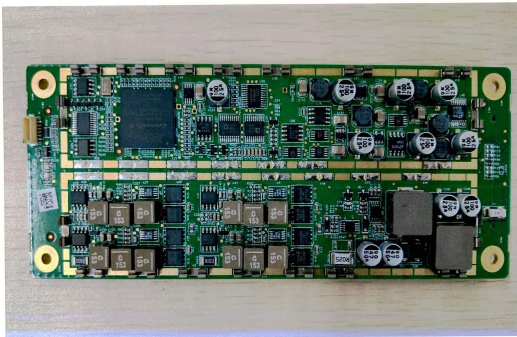
Плата 4D/TEE
