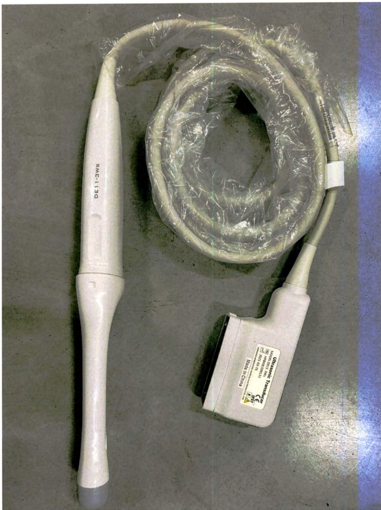
Датчик ультразвуковой объемный внутриполостной DE11-3Ws
