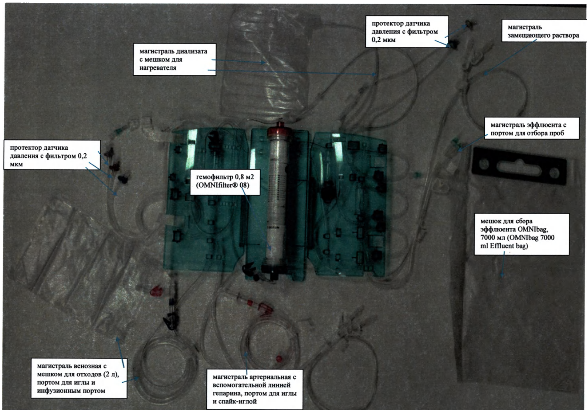
Рис.3. Набор кровопроводящих магистралей OMNiset®, включающий гемофильтр OMNIfilter® для гемодиализа однократный к аппарату для экстракорпоральной очистки крови OMNI®, вариант исполнения: Набор кровопроводящих магистралей OMNiset® 0,8 м 2 , включающий гемофильтр (OMNIfilter® 0,8 м 2 ), для CVVH, CVVHD, CVVHDF и SCUF терапии. Состав.
