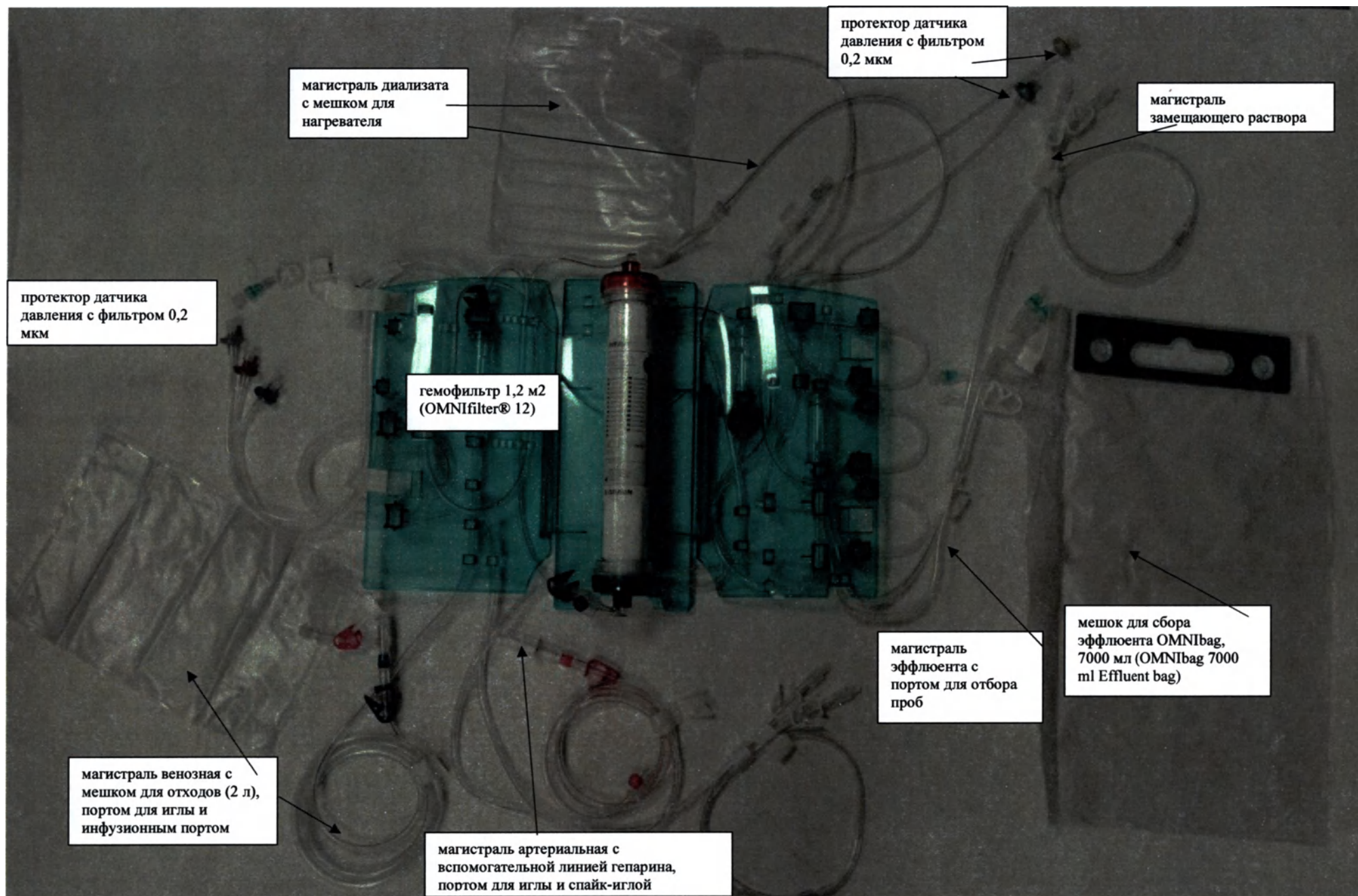
Рис.7. Набор кровопроводящих магистралей OMNIsat® 1,2 м², включающий гемофильтр (OMNIfilter® 1,2 м²), для CVVH, CVVHD, CVVHDF и SCUF терапии. Состав
