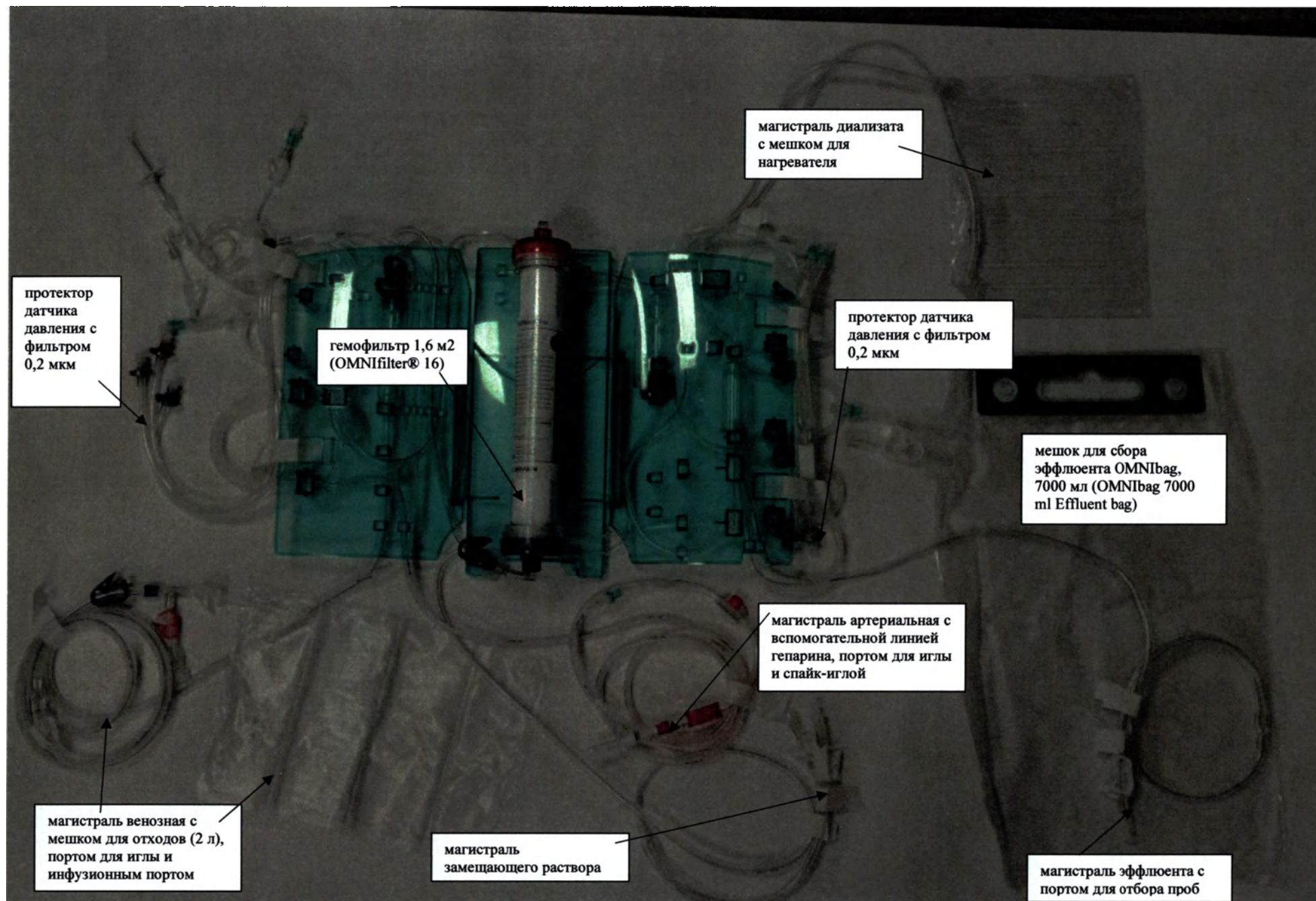
Рис. 23. Набор кровопроводящих магистралей OMNiset® Pro 1,6 м2 с гемодиализным гемофильтром (OMNIfilter® 1,6 м2), для CVVHD, CVVHDF и SCUF терапии. Состав
