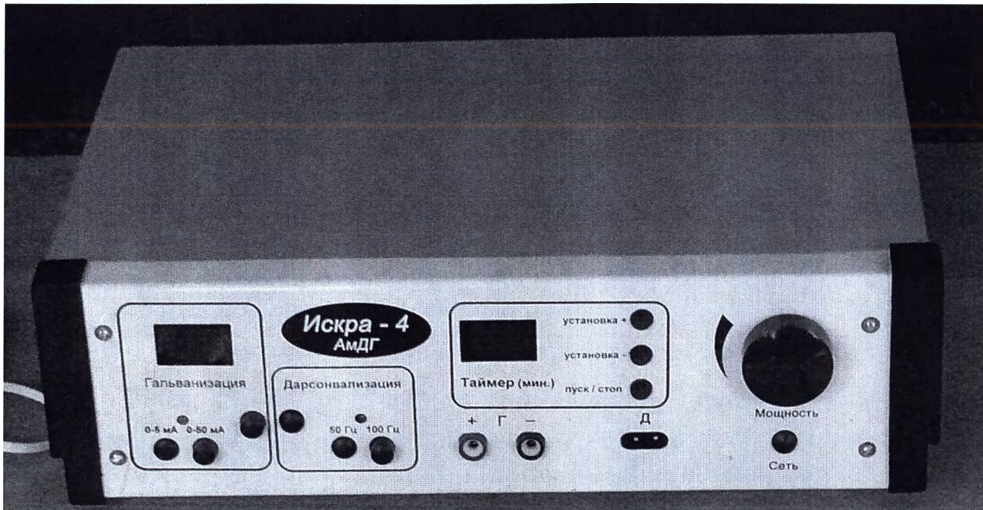
Внешний вид «Аппарат для местной дарсонвализации и гальванизации АмДГ-«Искра-4» по ТУ 9444-003-34711238-2005, исполнение 01.
