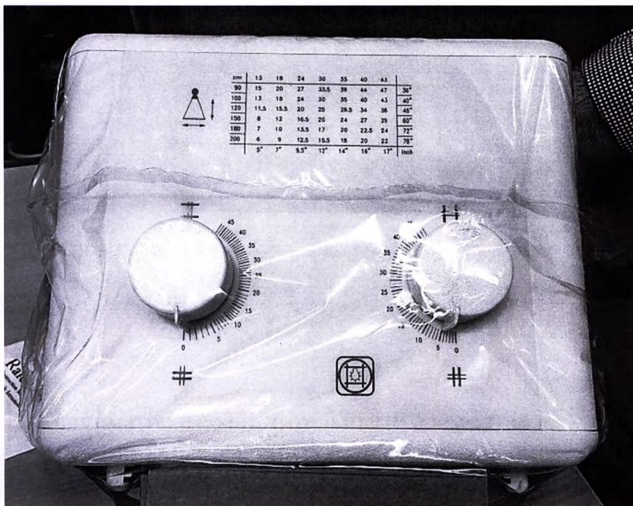
Коллиматор с соединительными элементами, с ручным управлением, серия R225 производства Ralco S.r.l, Италия
