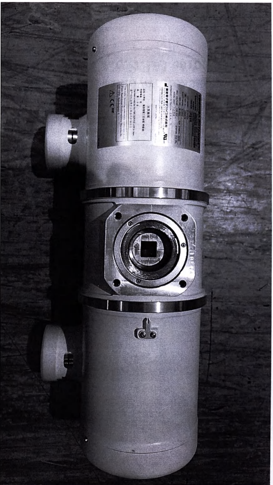
Излучатель рентгеновский с рентгеновской трубкой E7252X, или E7865X, или E7884X производства фирмы Canon Electron Tubes & Devices Co. Ltd., Япония
