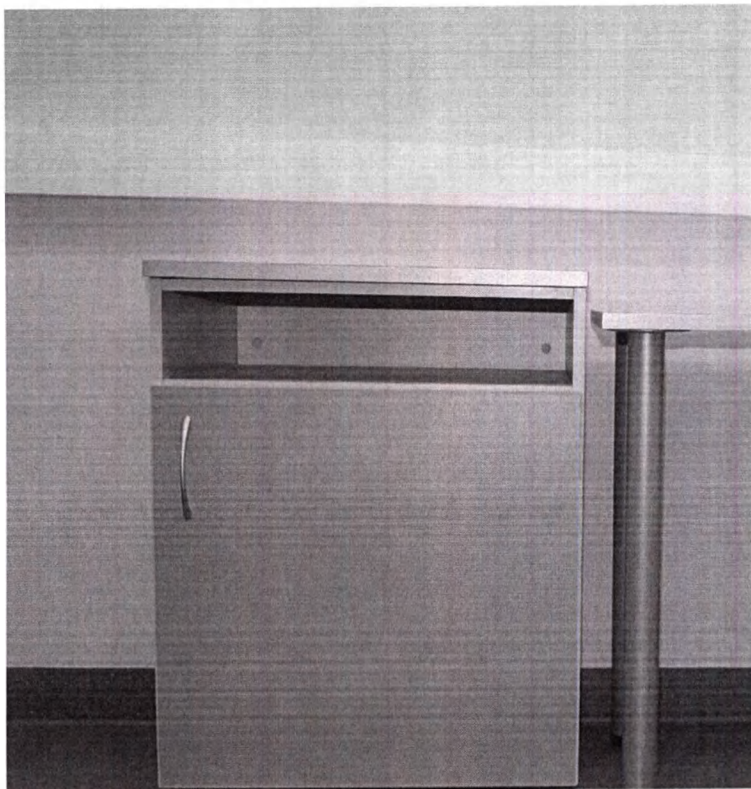
Фото 12 Тумба модель М-ТКн-40, М-ТКн-50, М-ТКн-60 общий вид
