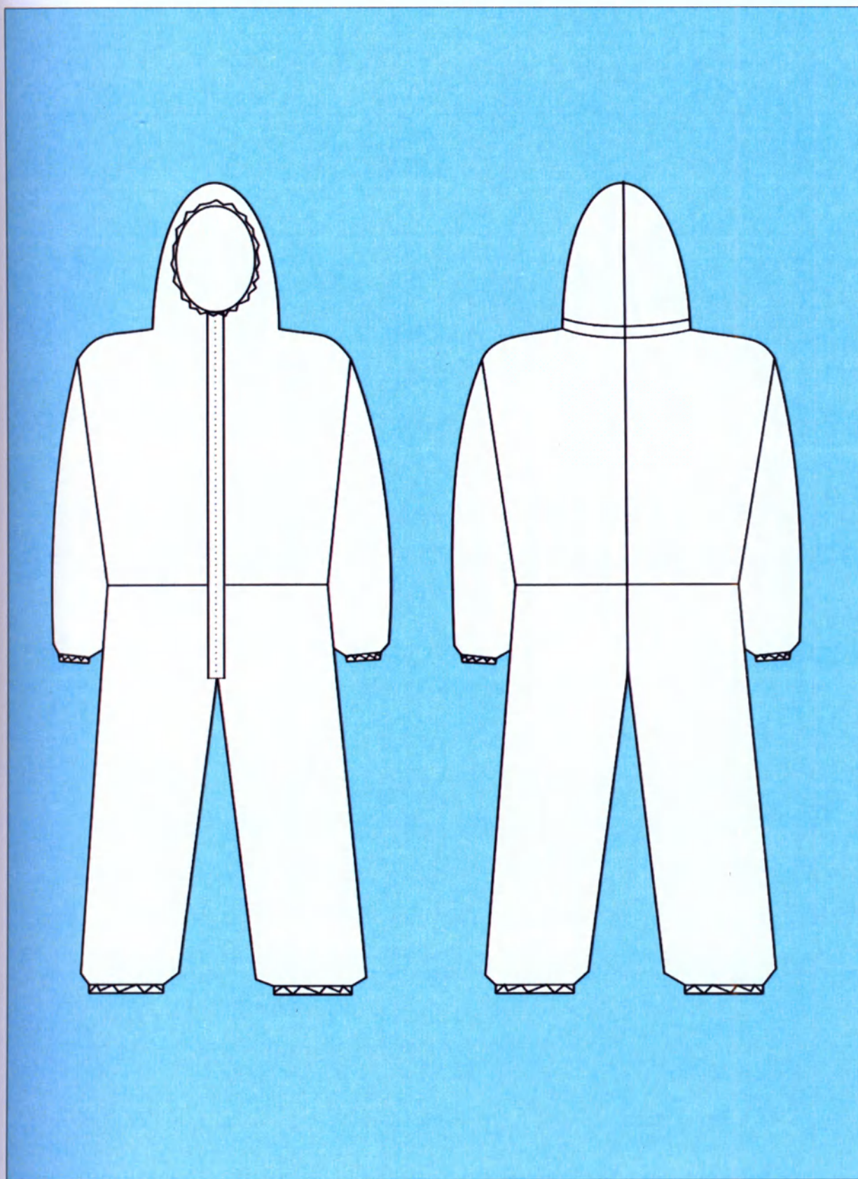
Костюм противоэпидемический одноразовый на молнии (технический рисунок)
