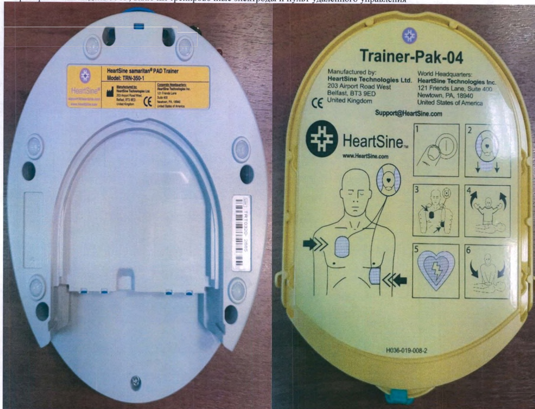
6. Тренировочная модель 350P, включая тренировочные электроды и пульт удаленного управления
