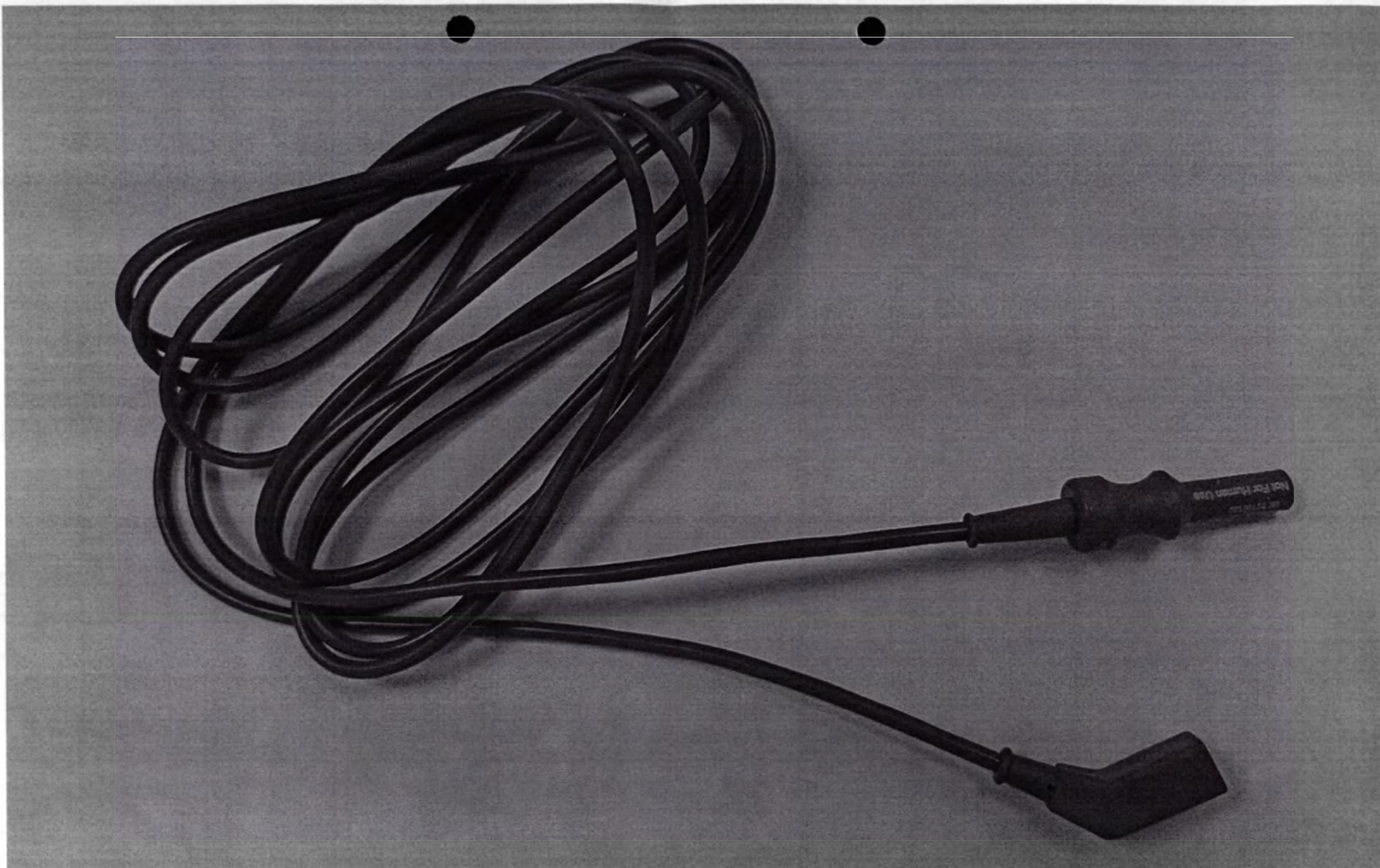
Штекер Aescular для щипцов - штекер совместимый с генератором Martin, Berchtold, Aescular GK55, GK60, 3 м, 80100130 Данный внешний вид также актуален для варианта исполнения - штекер совместимый с генератором Martin, Berchtold, Aescular GK55, GK60, 5 м, 80100131. Отличие только в длине.
