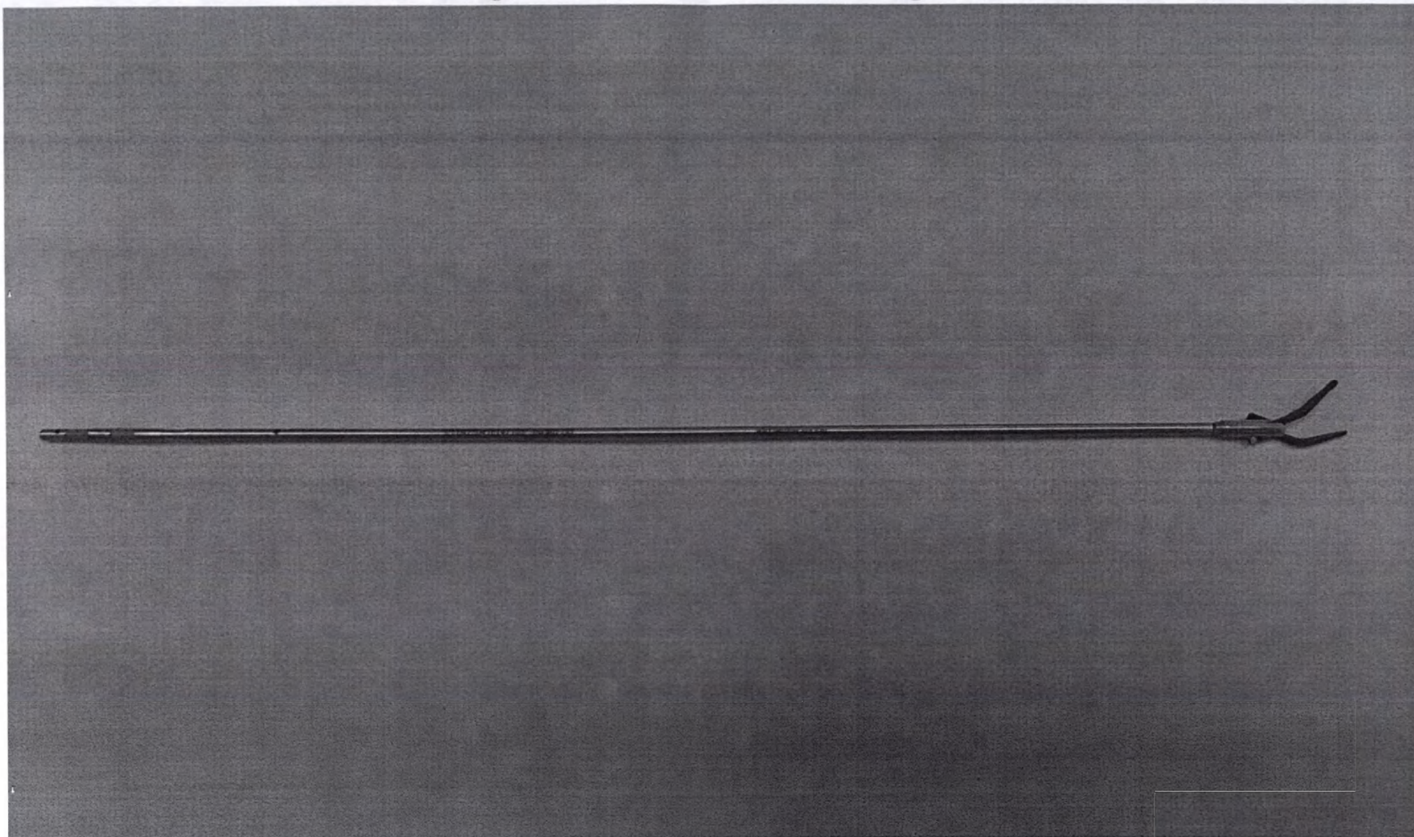
Электрод - вставка биполярный Mithras в виде щипцов типа Фламинго вертикальных, 30°, диаметр 1,2 мм, 82460346
