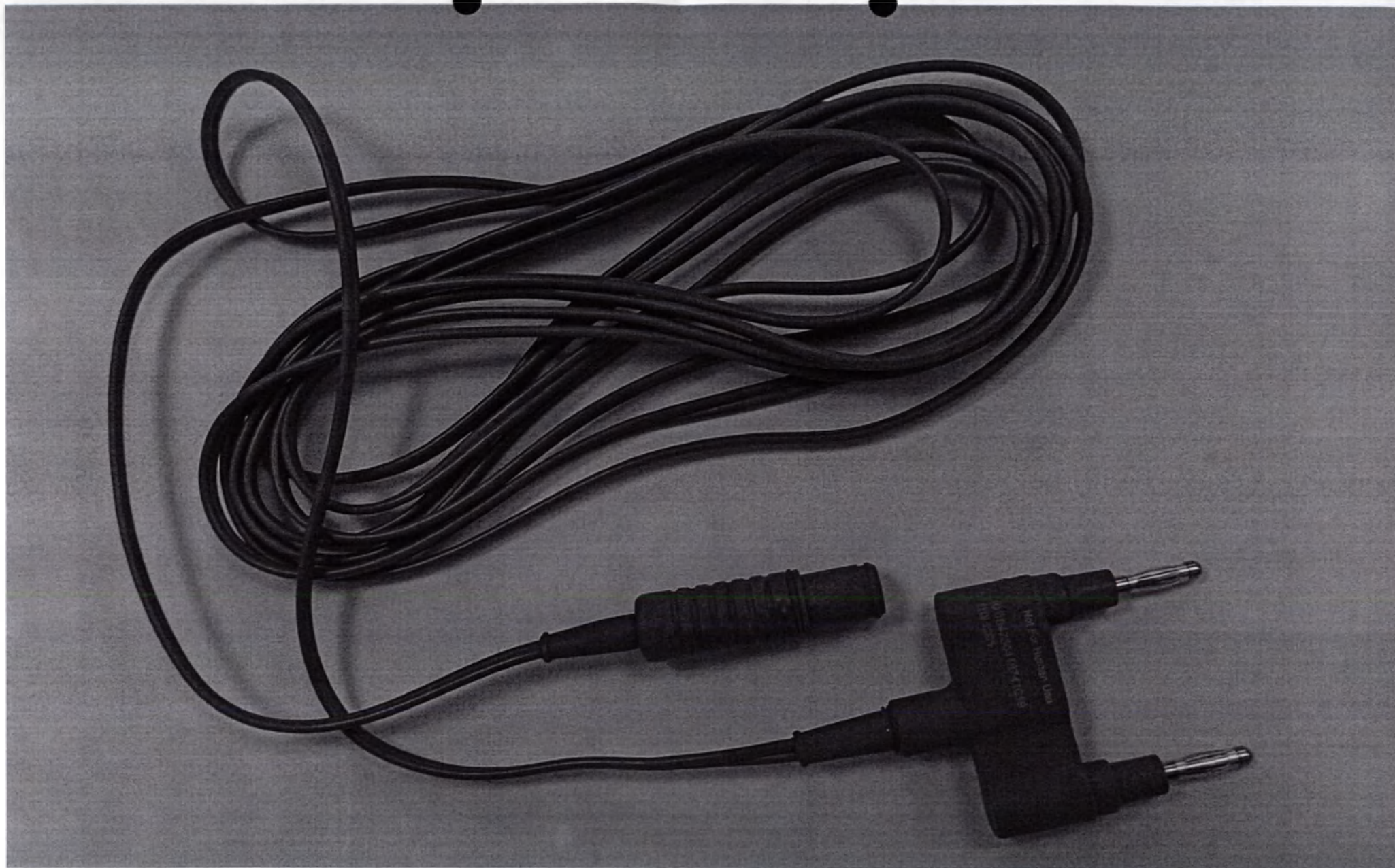
Штекер Karl Storz для щипцов - штекер U-20, 4 м, 80100268
