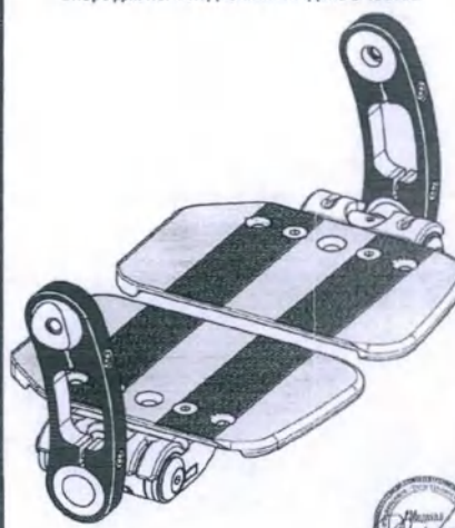
Опора для ног с подножкой Модель 3 403602
