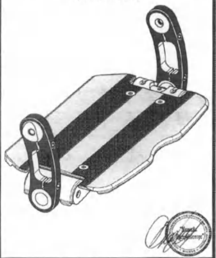
Опора для ног с подножкой Модель 2 внутреннее крепление 403902
