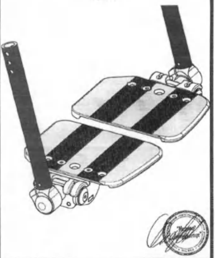
Опора для ног с подножкой Модель 4 внешнее крепление 404005
