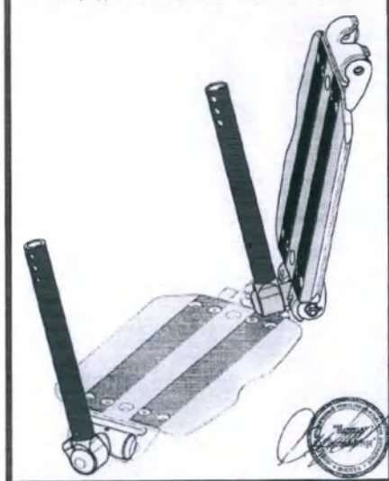
Опора для ног с подножкой Модель 5 403611
