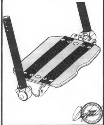
Опора для ног с подножкой Модель 2 внешнее крепление 404002
