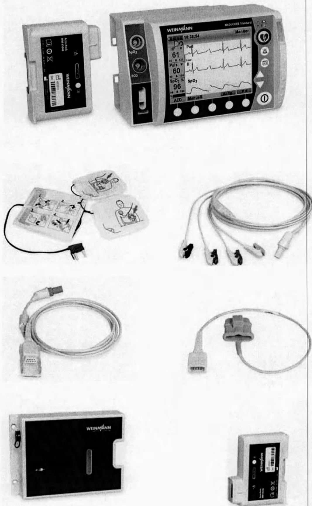
Портативный аппарат для электроимпульсной терапии и мониторингирования состояния пациента «MEDUCORE Standard» с принадлежностями
