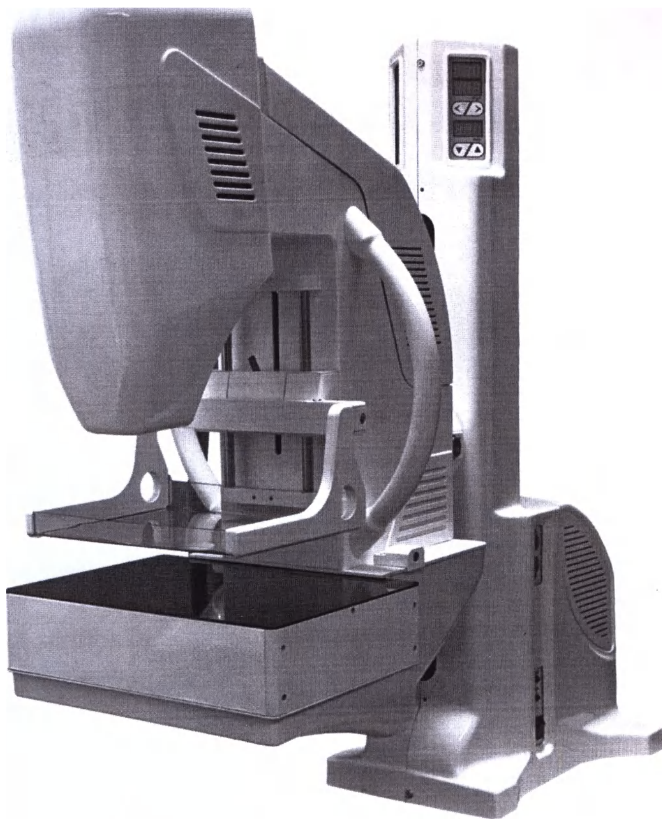
Рисунок 1 - Комплекс рентгеновский маммографический цифровой МАДИС ТУ У 33.1-14309534-118-2003. Устройство рентгеновское штативное со встроенной рентгеновской трубкой 0,006БД24-45
