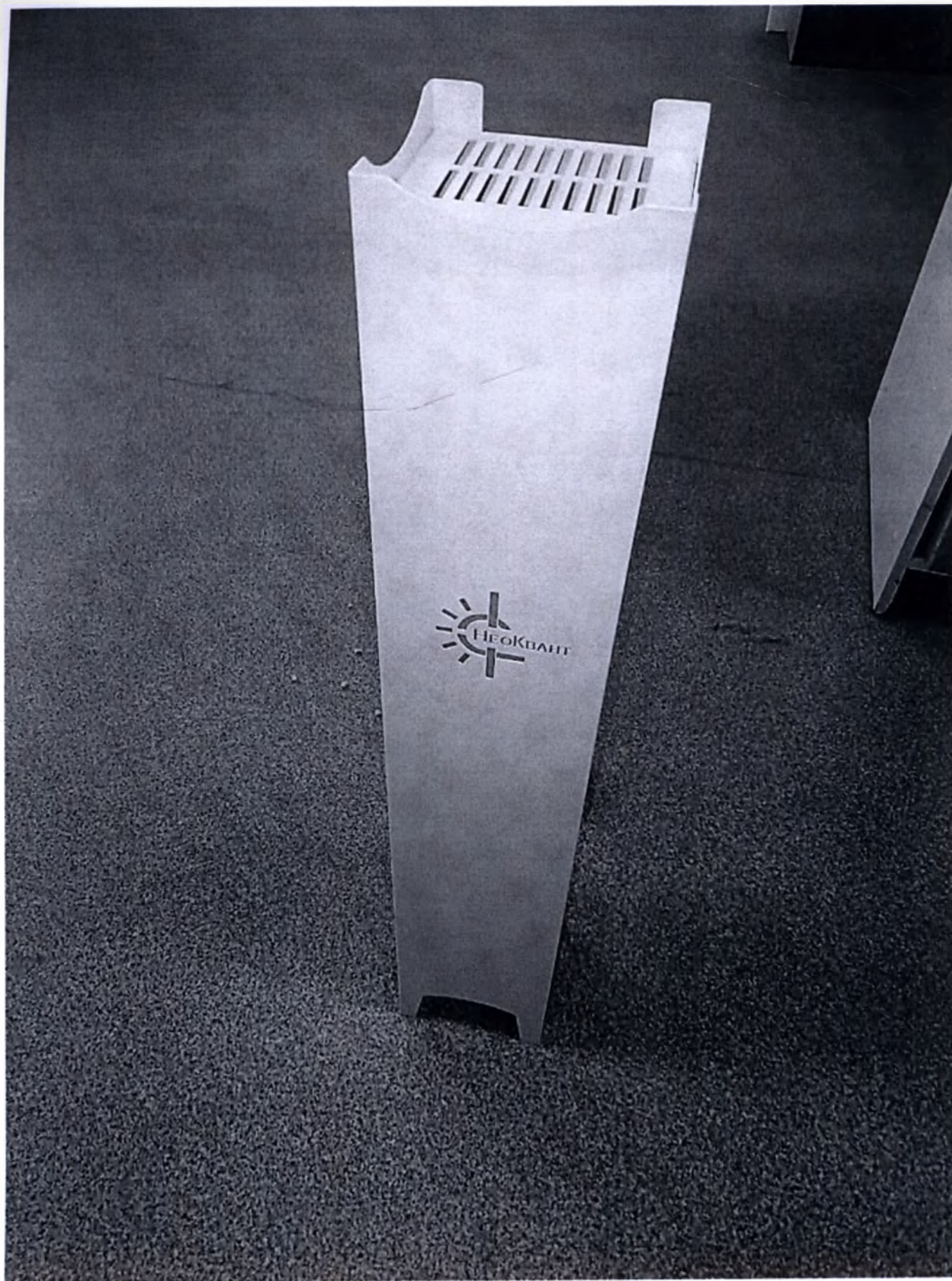
Общий вид Облучателя-рециркулятора ультрафиолетового закрытого типа «НеоКвант-РБ 30» и «НеоКвант-РБ 30С»
